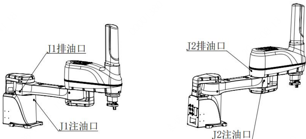
图 4-1 机器人油口位置图
