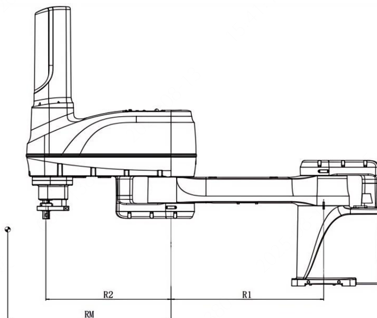
图 3-19 等效重量计算示意图
