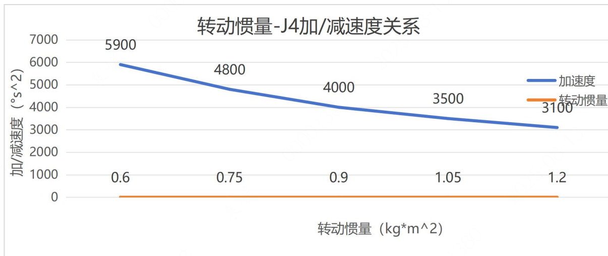
图 3-21 ESR30 系列负载转动惯量与四轴加速度关系曲线
