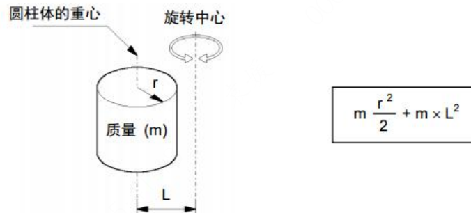
图 3-25 圆柱体的惯性力矩计算
