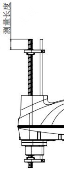
图 3-33 调整三轴的行程
