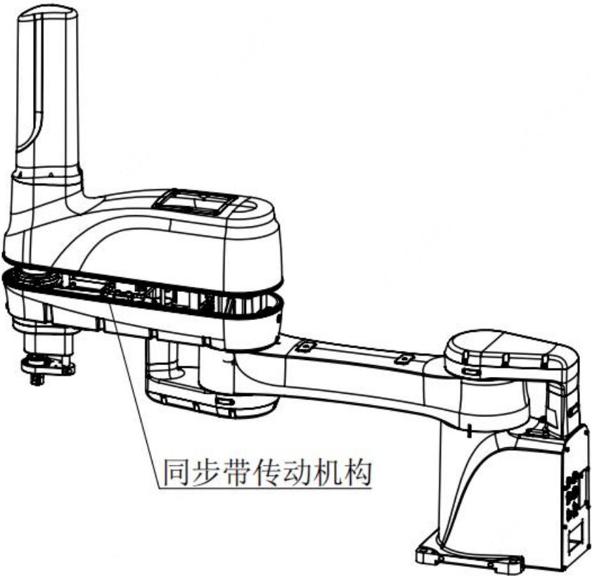
图 4-3 同步带传动机构示意图
