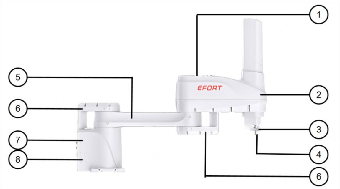
图 3-3 本体示意图
