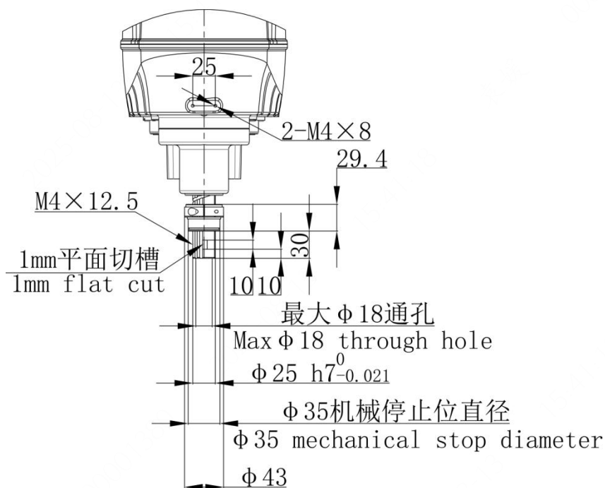
图 3-8 ESR20 系列工具安装接口尺寸
