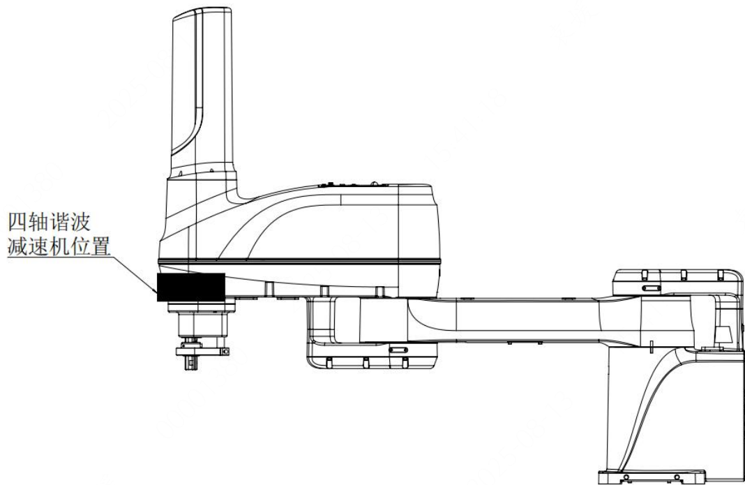
图 4-2 谐波减速机位置示意图
