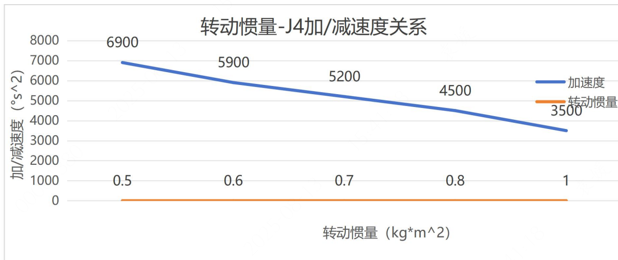
图 3-20 ESR20 系列负载转动惯量与四轴加速度关系曲线
