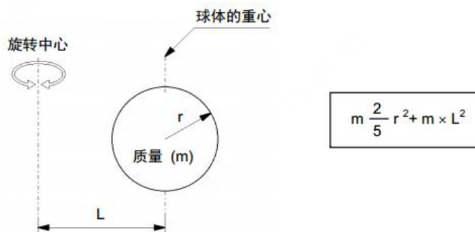
图 3-26 球体的惯性力矩计算
