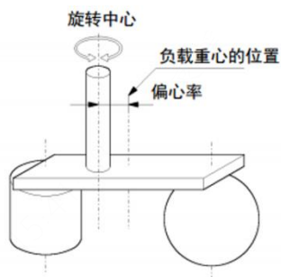
图 3-22 轴上安装负载的离心率(偏心率)示意图
