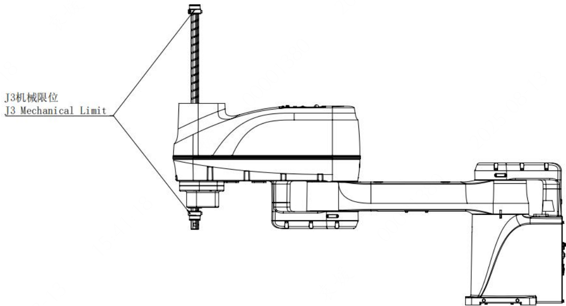
图 3-32 三轴机械限位位置示意图
