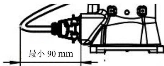
图 3-11 底座线缆后侧出线最小弯折尺寸
