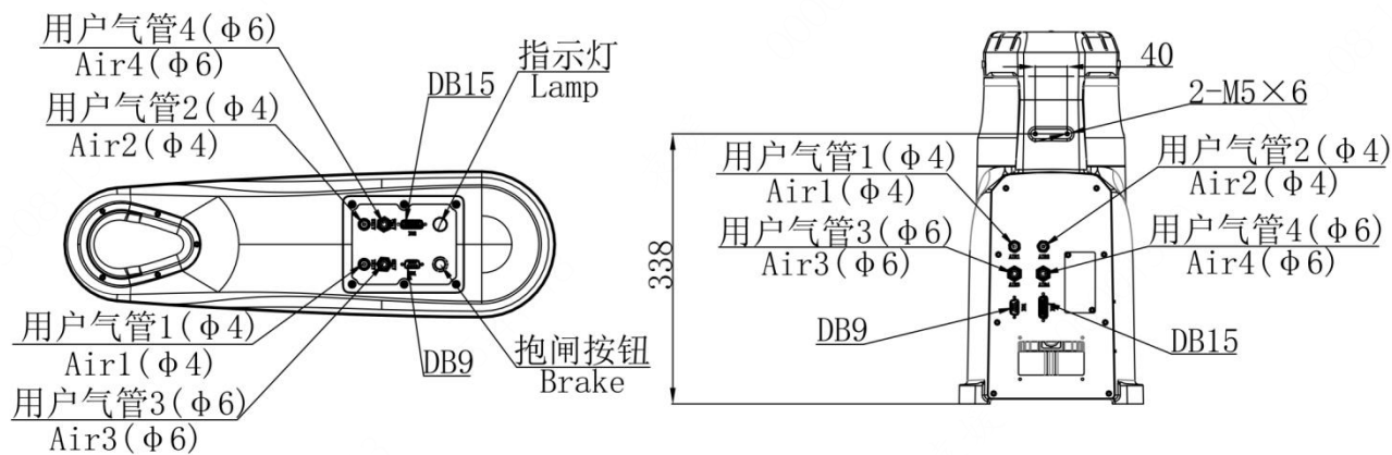
图 3-17 用户配线与配管
