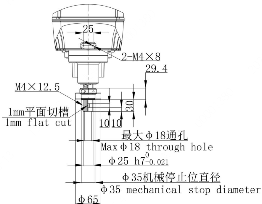
图 3-9 ESR30 系列工具安装接口尺寸
