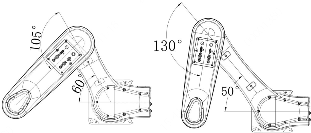
图 3-16 打包姿态示意图
