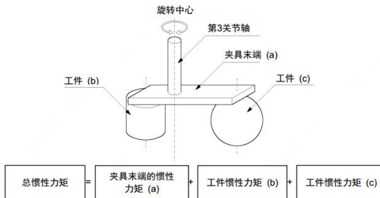
图 3-23 负载（握持工件的夹具末端）装载惯性（力矩）的计算
