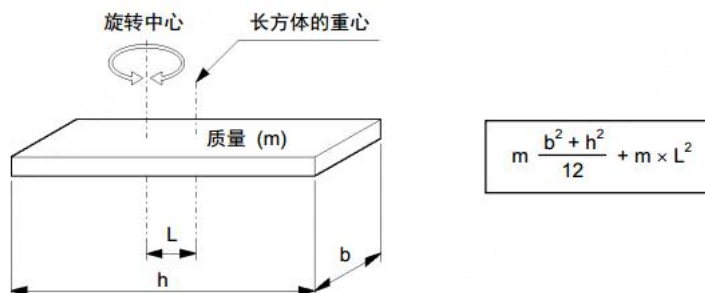
图 3-24 长方体的惯性力矩计算
