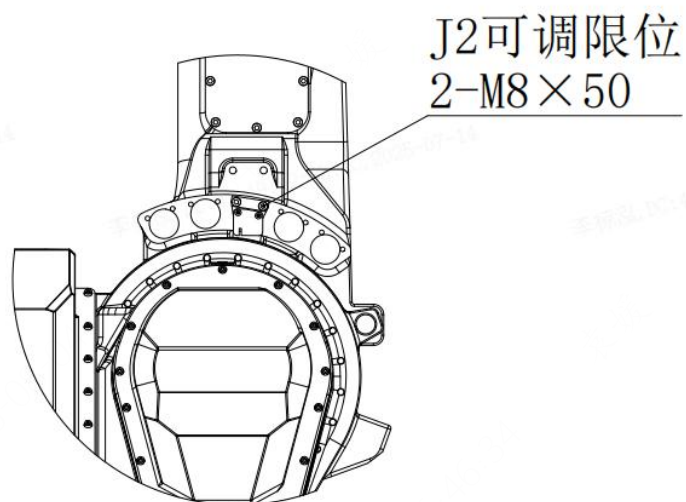
图 2-6 J2 轴可调限位图
