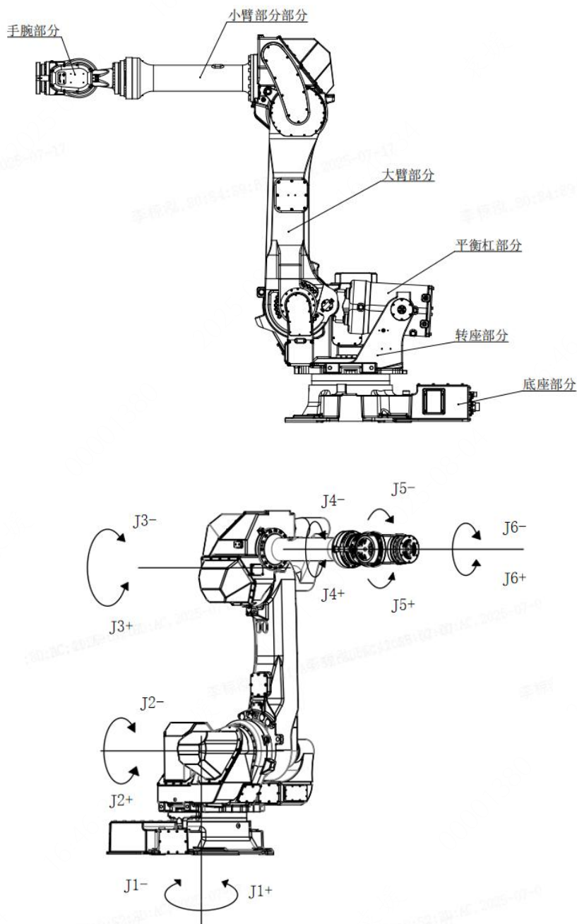
图 2-3 EXR210-2700 机械本体组成部分及各轴方向标识
