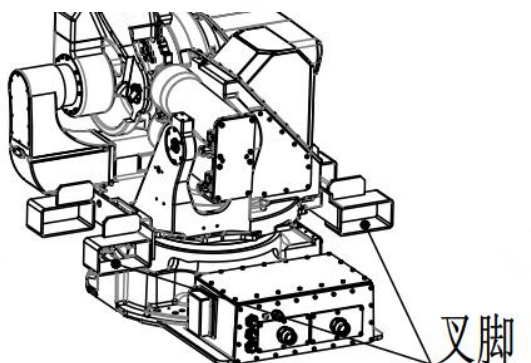
图 3-2 叉脚安装示意图
