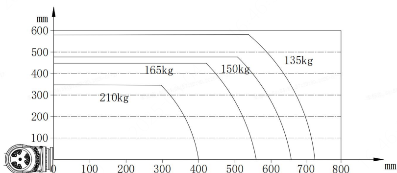
图 2-8 EXR210-2700 手腕轴转矩图
