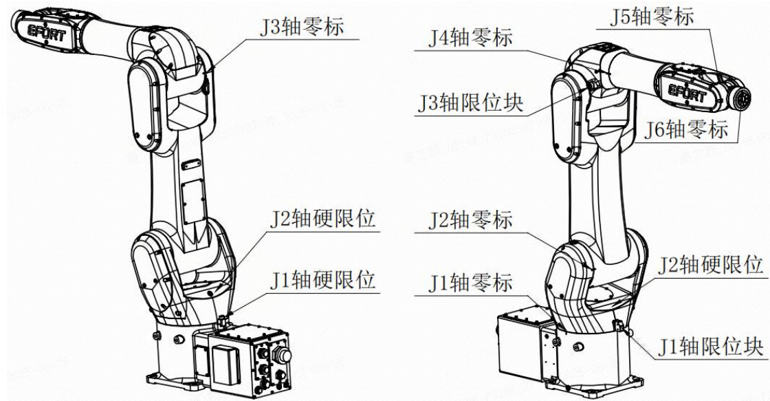
图 2-4 机械硬限位位置及零标位置
