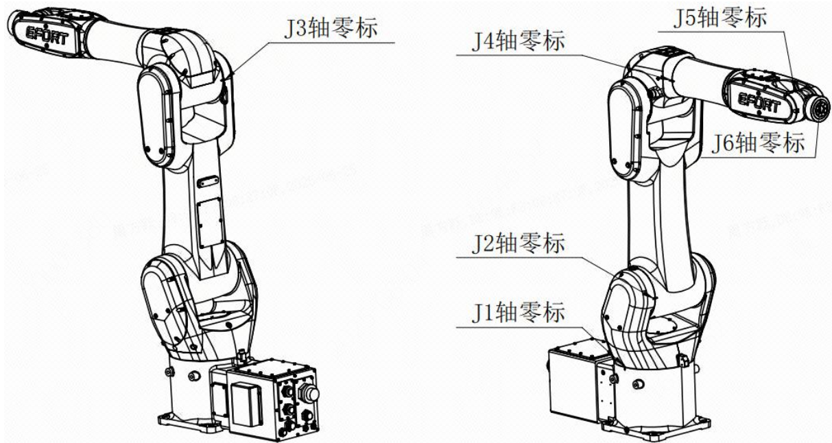
图 4-3 机器人零点位置图
