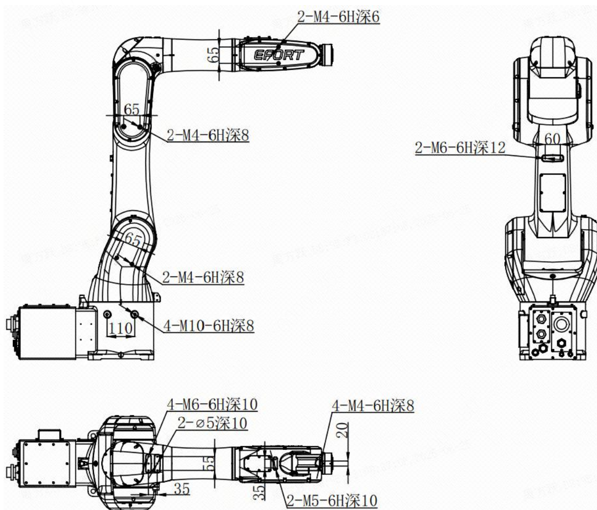
图 3-8 外围安装尺寸图
