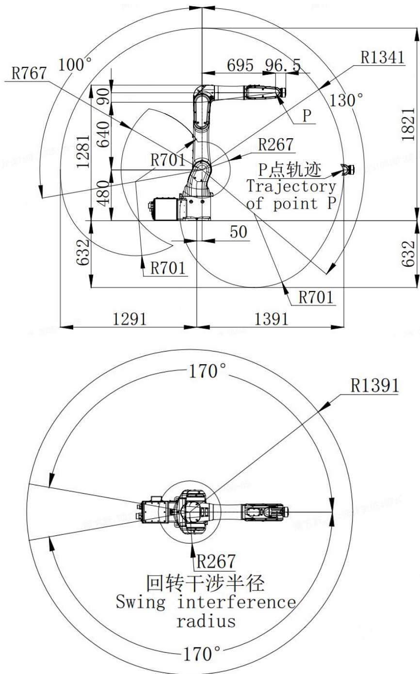
图 2-5 机器人工作空间图
