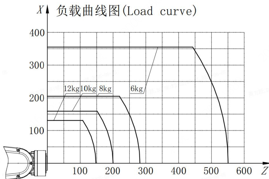
图 2-6 EXR12-1400 手腕轴转矩图
