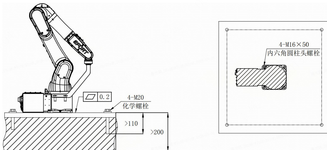
图 3-5 机器人安装举例
