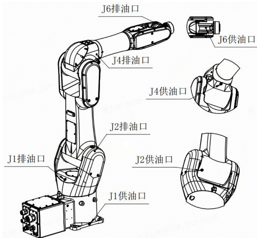
图 4-1 机器人注油口和排气口分布图
