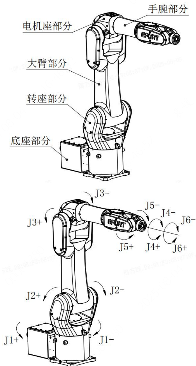
图 2-3 EXR12-1400 机械本体组成部分及各轴方向标识
