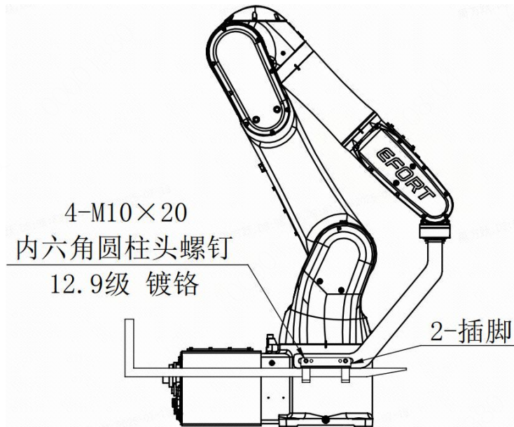
图 3-2 叉车搬运示意图
