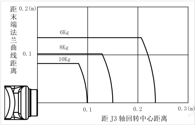
图 2-9 ER10-3-900 手腕轴转矩图
