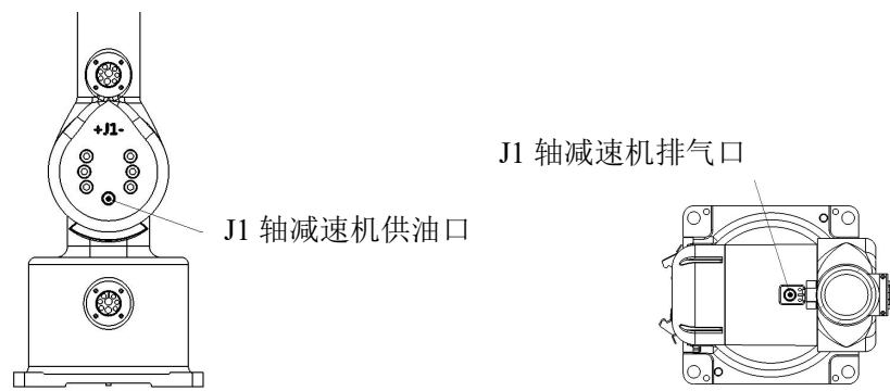
图 4-1 机器人注油口和排气口分布图
