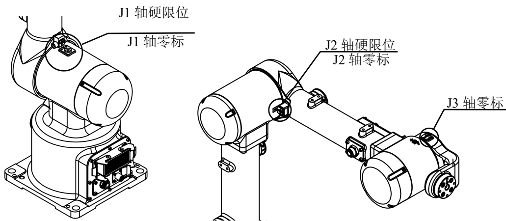
图 2-5 ER10-3-900 机械硬限位位置及零标位置
