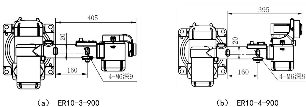
图 3-12 小臂杆上安装外部件尺寸图
