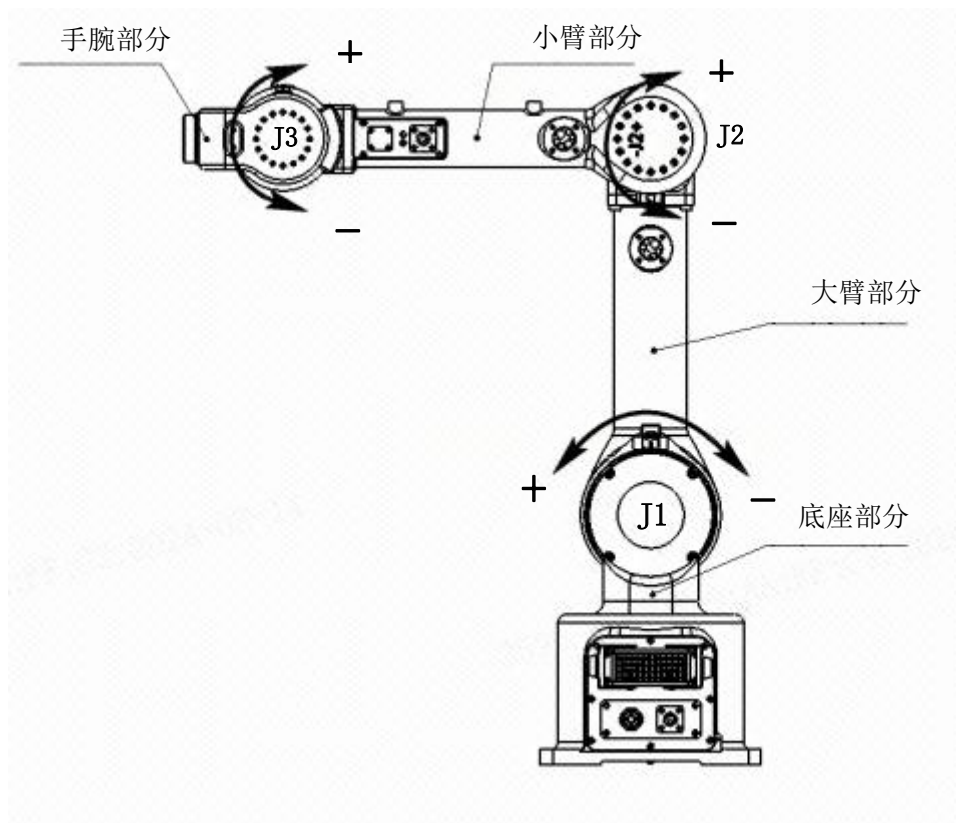
图 2-3 ER10-3-900 机械本体组成部分
