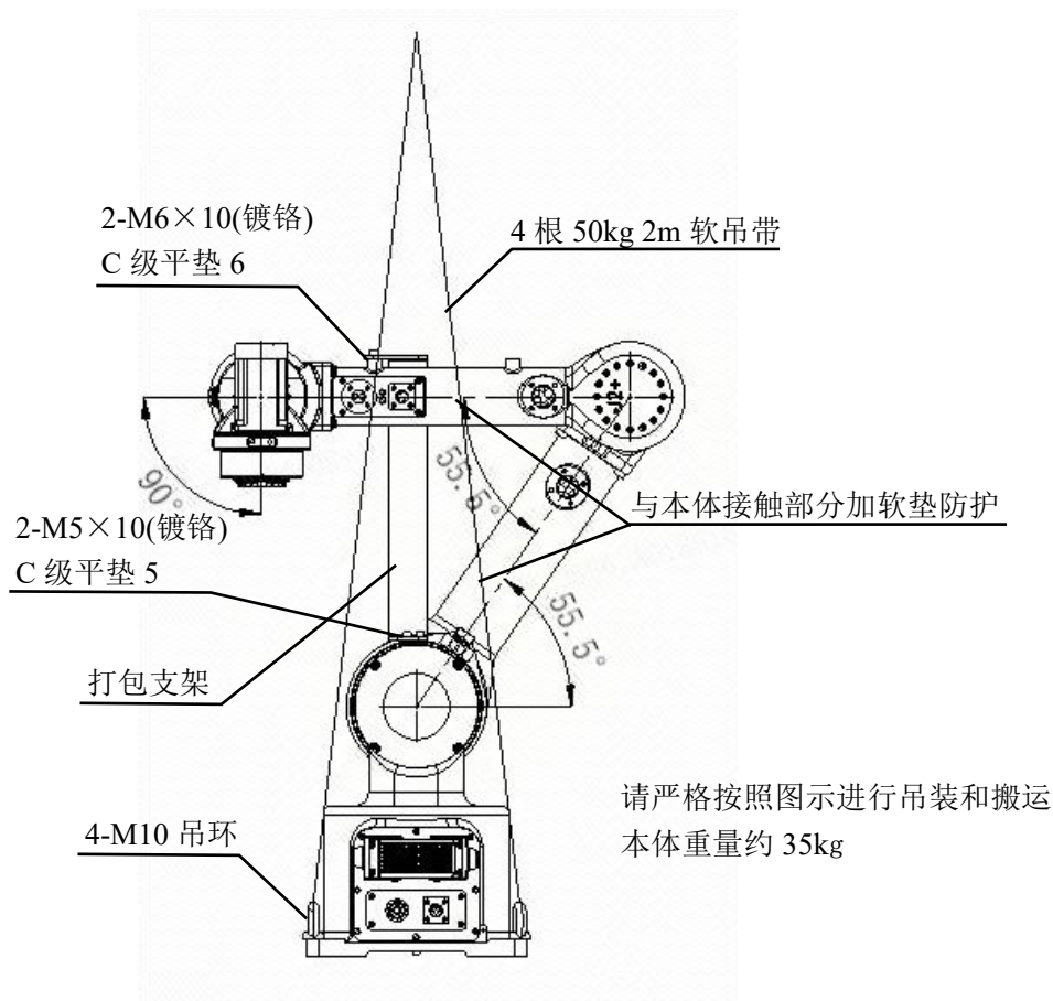
图 3-5 ER10-4-900 吊装搬运示意图
