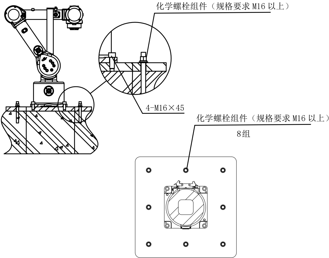
图 3-8 机器人安装举例
