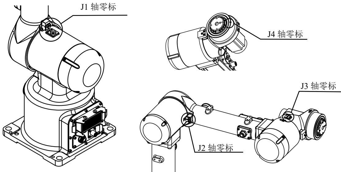
图 4-5 ER10-4-900 机器人零点位置图
