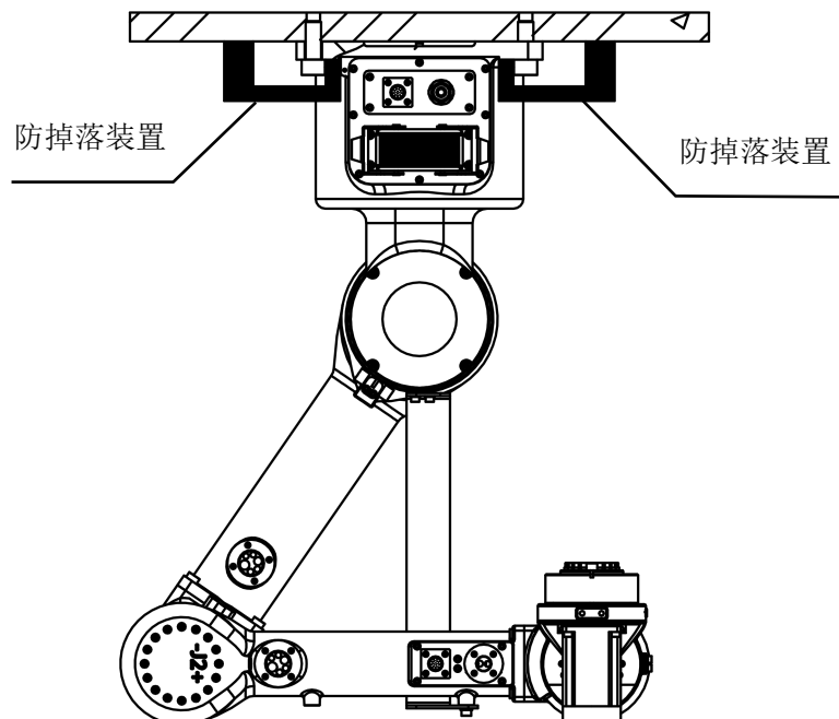
图 3-9 倒挂安装
