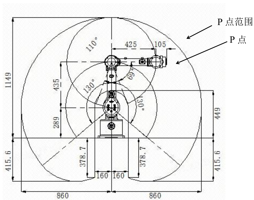
图 2-8 ER10-4-900 机器人工作空间图
