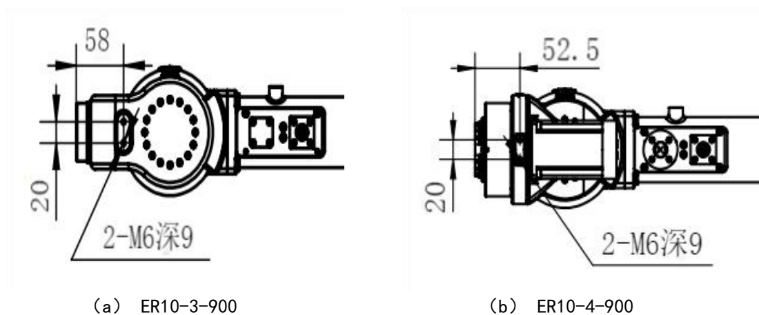
图 3-13 手腕体上安装外部件尺寸图
