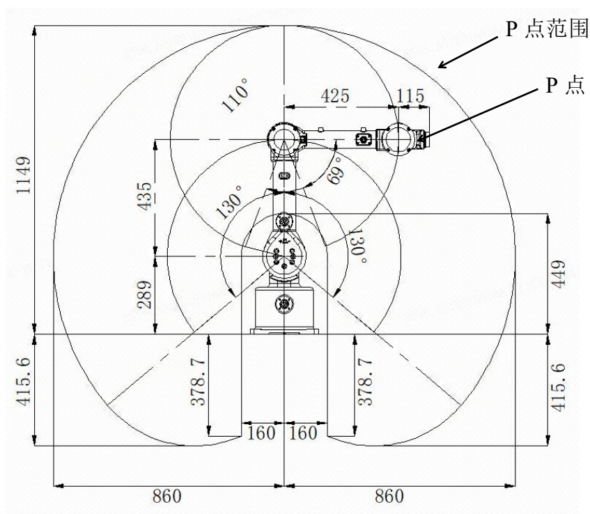
图 2-7 ER10-3-900 机器人工作空间图
