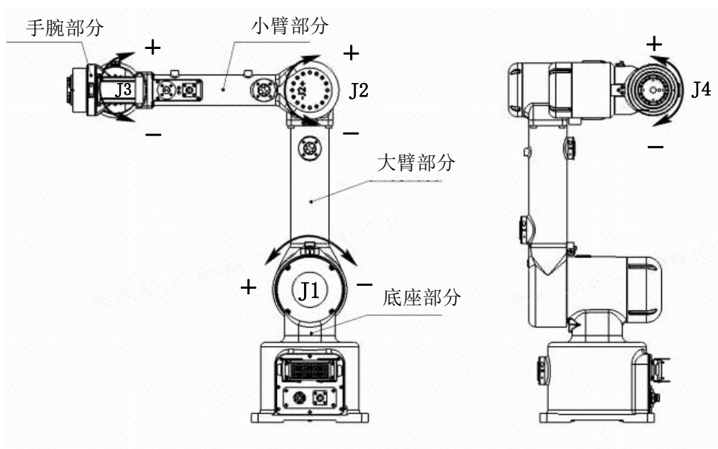
图 2-4 ER10-4-900 机械本体组成部分
