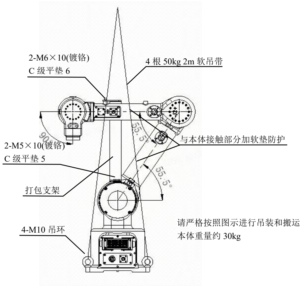
图 3-4 ER10-3-900 吊装搬运示意图
