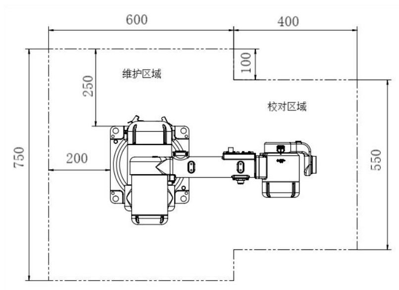
图 4-2 ER10-3-900 维护及使用区域
