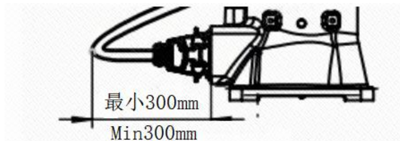
图 3-7 底座线缆后侧出线最小弯折尺寸
