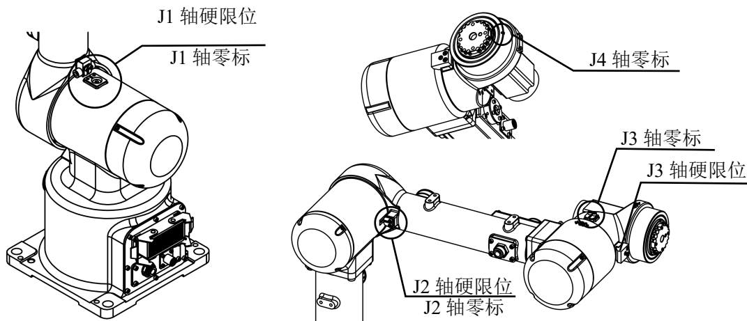
图 2-6 ER10-4-900 机械硬限位位置及零标位置
