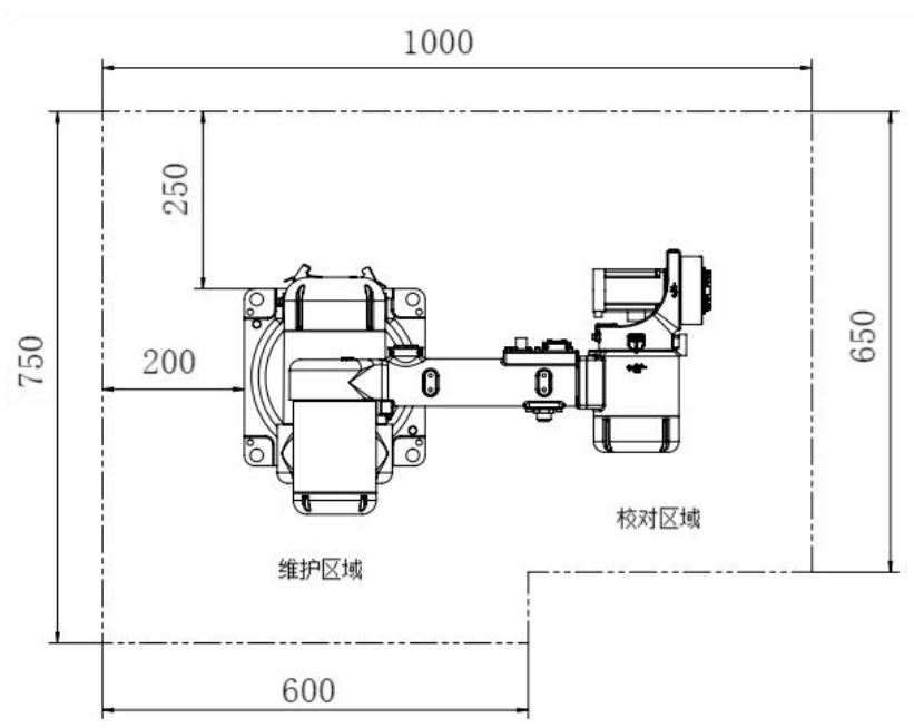
图 4-3 ER10-4-900 维护及使用区域
