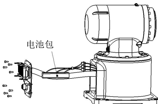
图 4-6 机器人电池组位置图
