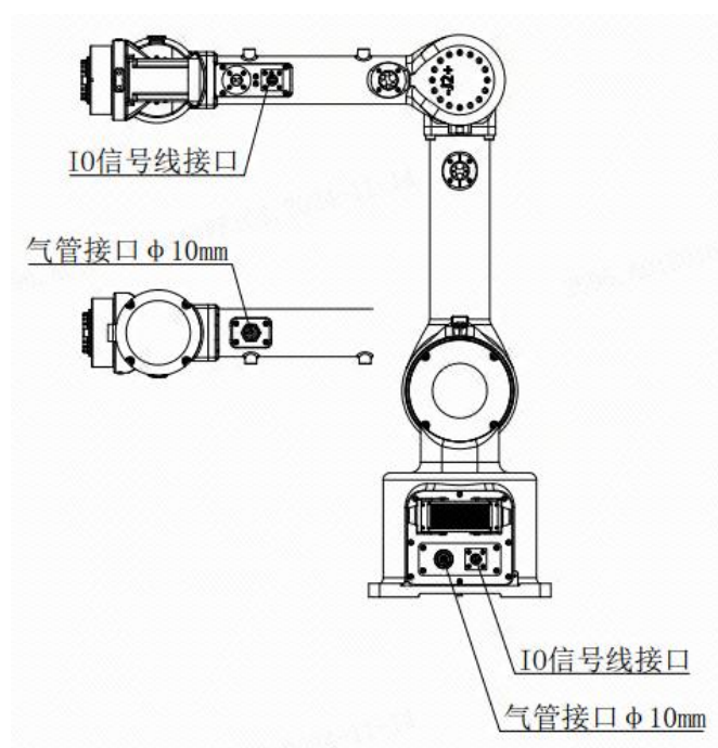
图 3-14 气路及信号线接口位置
