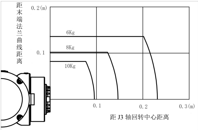
图 2-10 ER10-4-900 手腕轴转矩图
