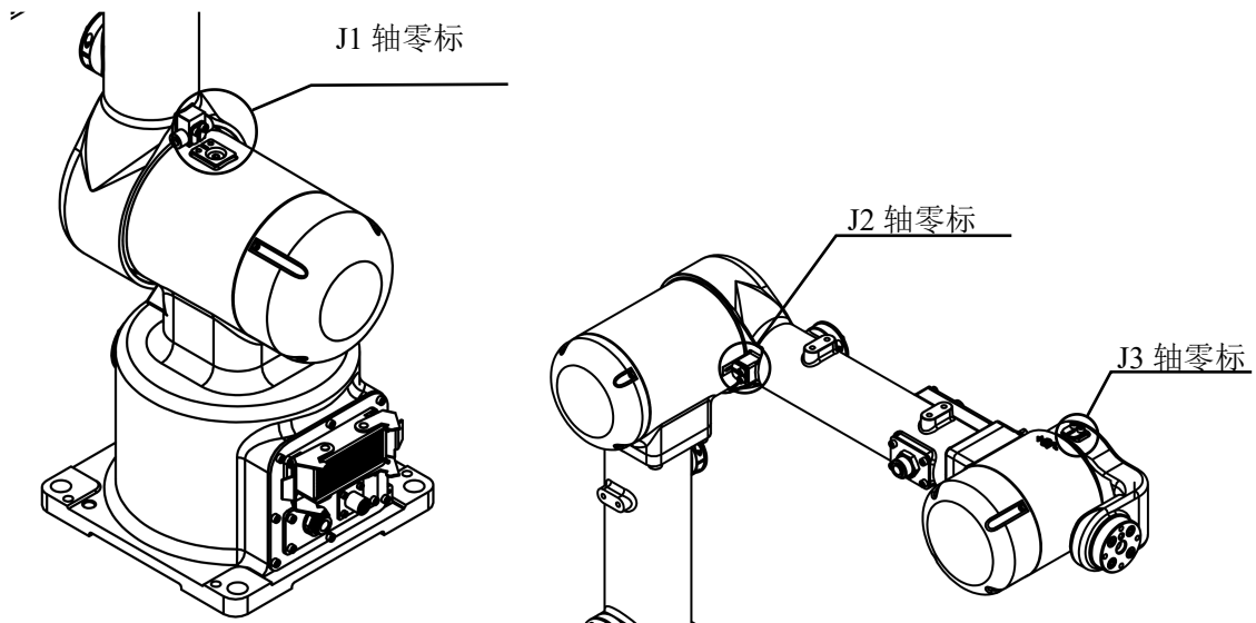
图 4-4 ER10-3-900 机器人零点位置图
