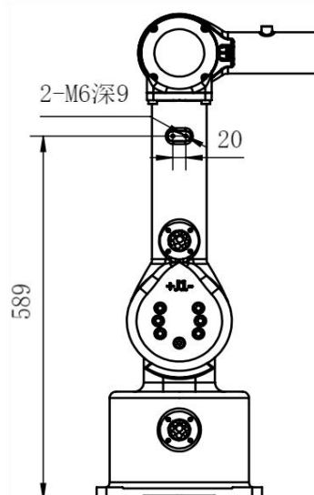
图 3-11 ER10-3(4)-900 大臂上安装外部件尺寸图
