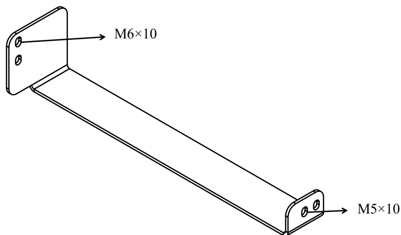
图 3-1 打包固定支架示意图
