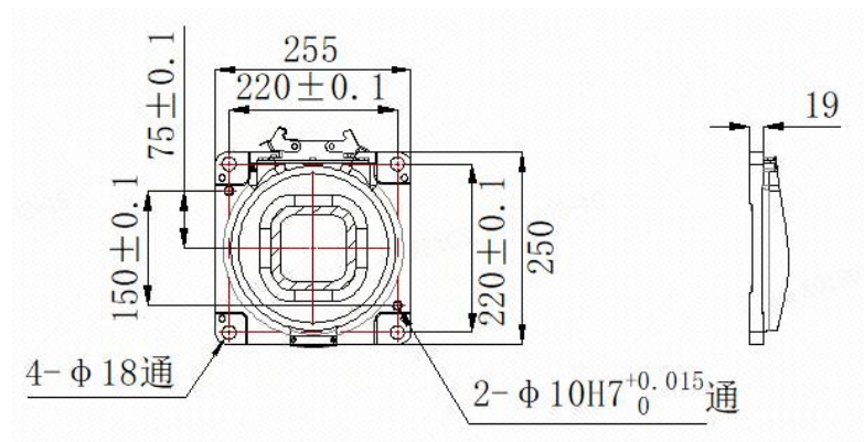
图 3-6 机器人底座尺寸
