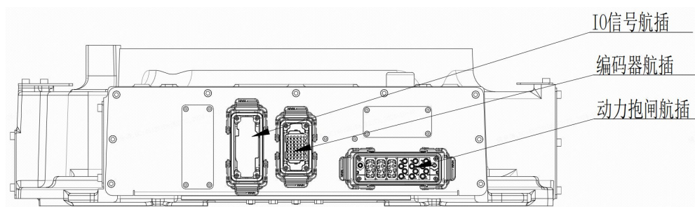
图 3-14 底座部分信号线接口
