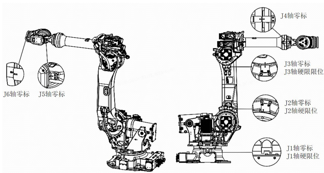
图 2-6 各轴零标及硬限位示意图
