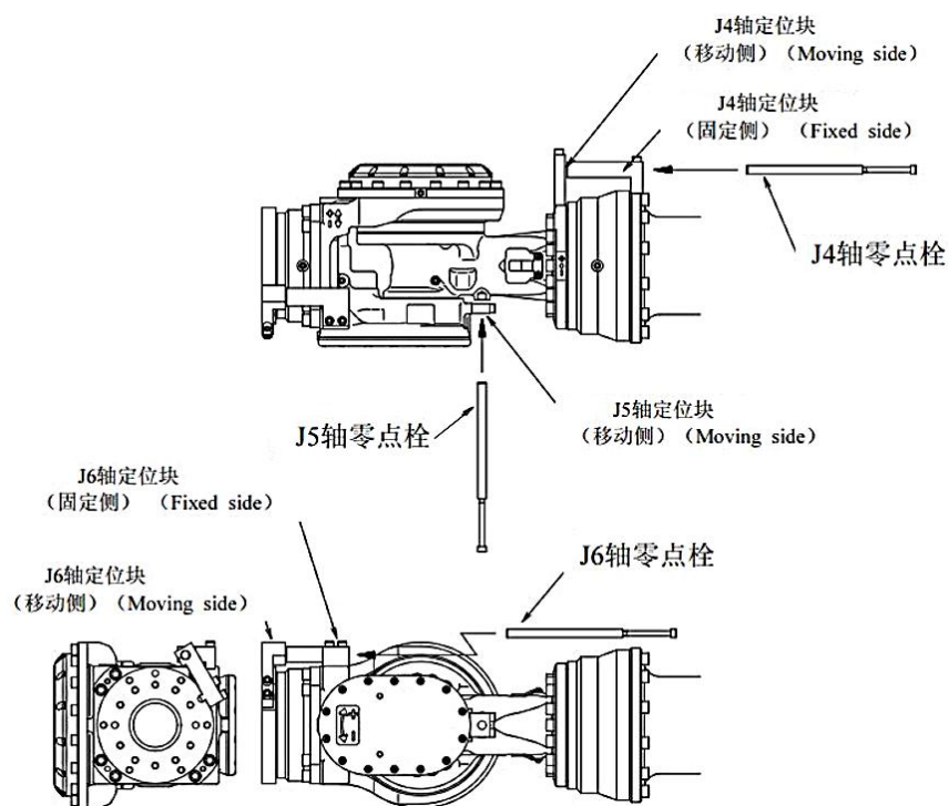
图 4-4 ER210-2700 V2 零点位置图
