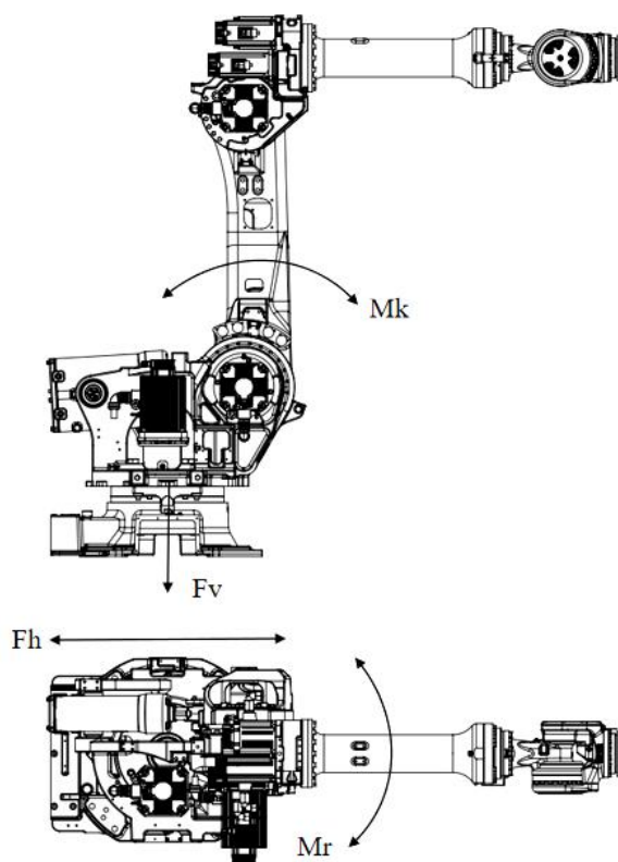
图 3-7 机器人底座受力图
