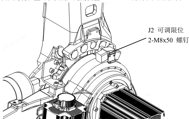
图 2-8 J2 轴可调限位图
