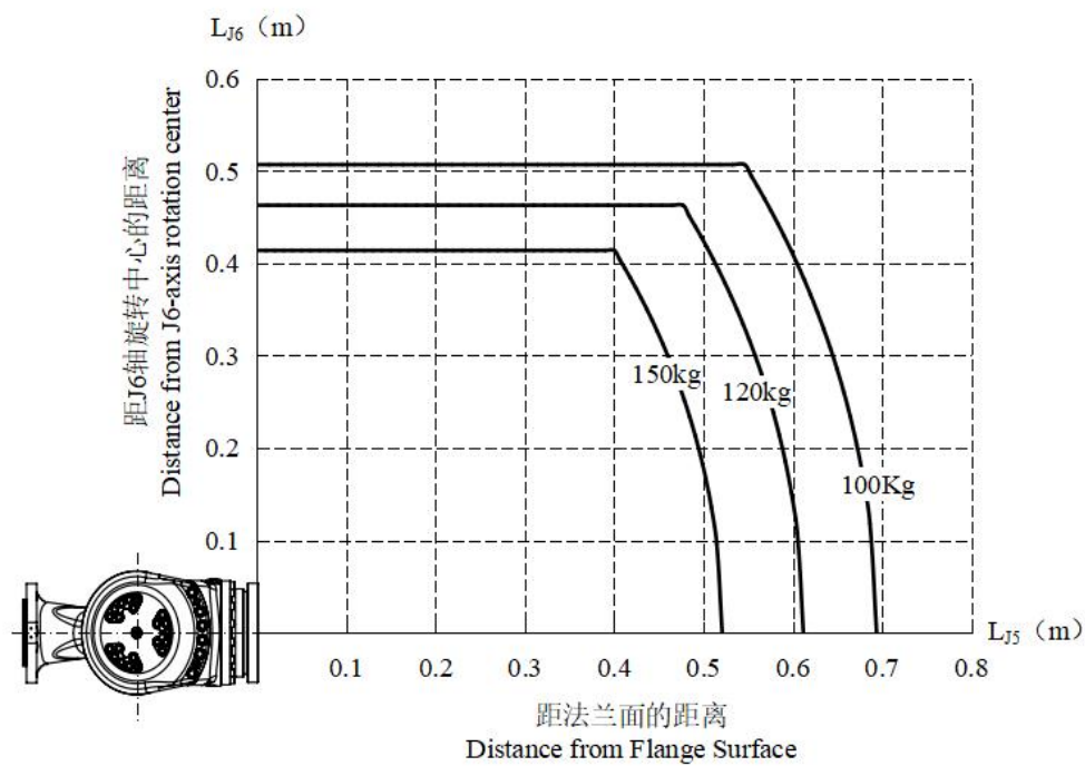
图 2-9 ER150-2700 手腕轴扭矩图
