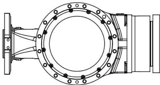
图 2-1 210-2700 V2 手腕示意图
