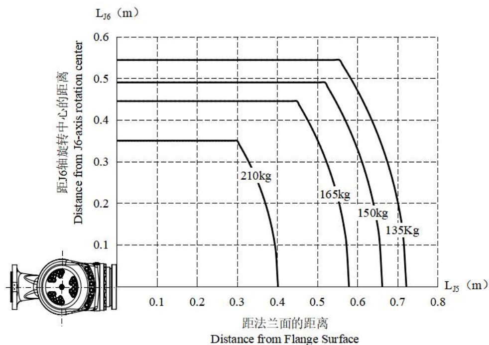
图 2-8 ER210-2700 手腕轴扭矩图
