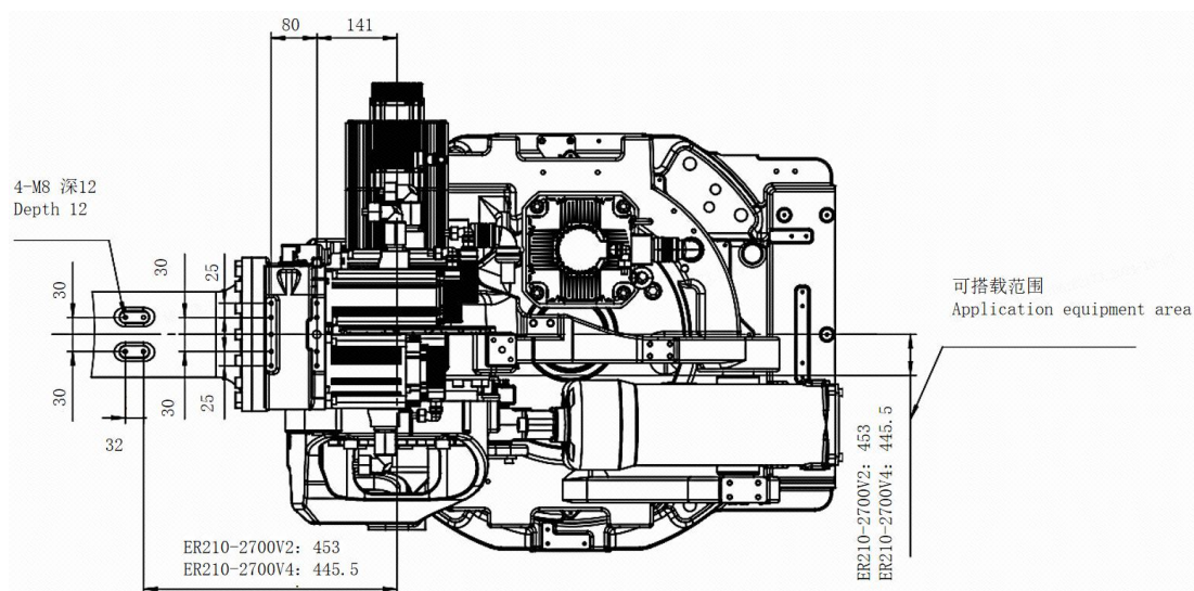
图 3-10 电机座/小臂杆上安装外部件尺寸图
