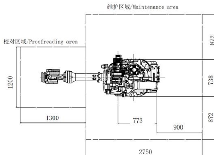
图 4-3 机器人维护及使用区域
