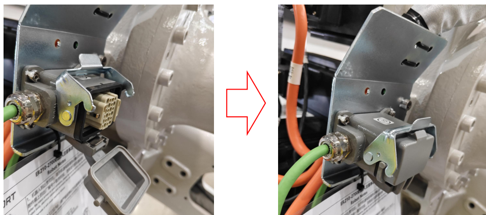
图 3-13 IO 接头安装示意图
