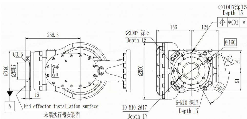
图 3-8 ER210-2700 V2 末端负载安装法兰尺寸及末端负载安装尺寸
