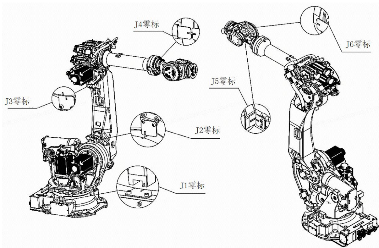
图 4-5 ER210-2700 V4 及 ER150-2700 零点位置图
