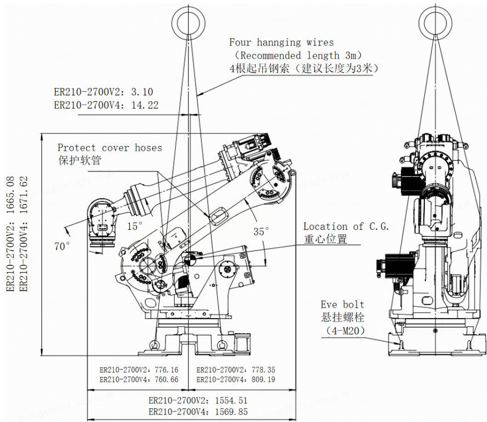
图 3-3 吊装搬运示意图 (ER150-2700 与 ER210-2700 V4 相同)
