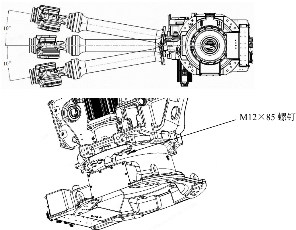
图 2-7 J1 轴可调限位图
