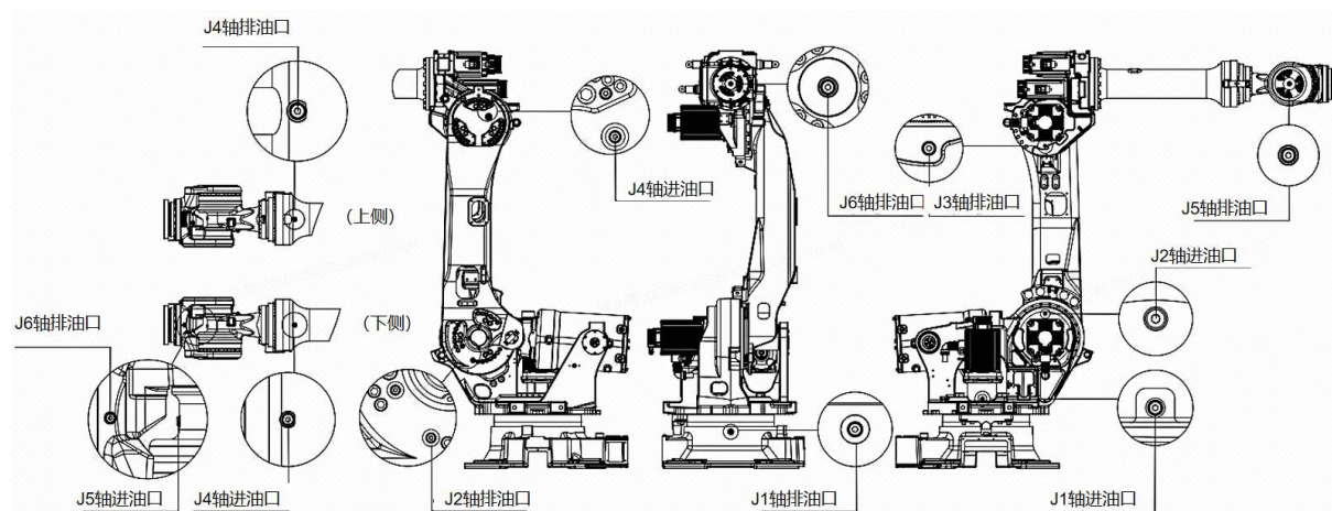
图 4-2 ER210-2700 V4 及 ER150-2700 供脂口和排气口分布图
