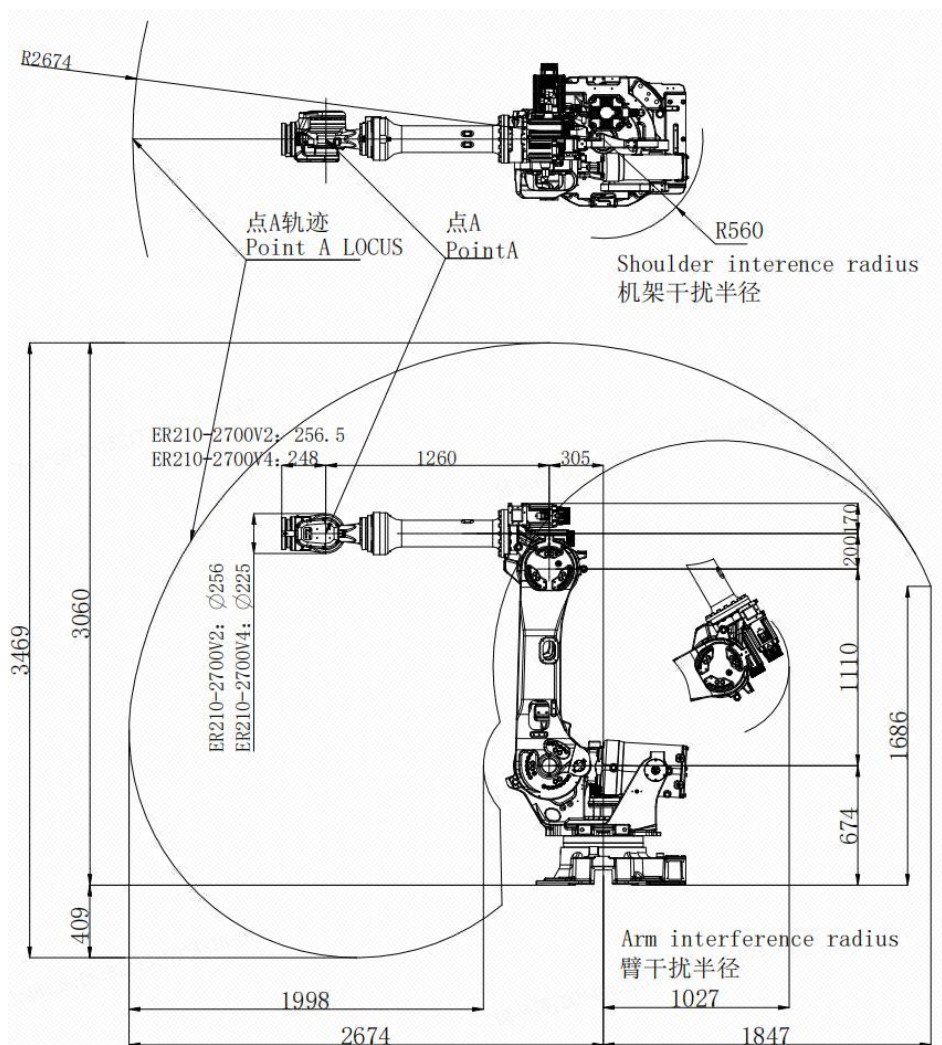
图 2-7 机器人运动范围图 (ER150-2700 与 ER210-2700 V4 相同)
