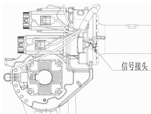
图 3-15 小臂部分信号线接口
