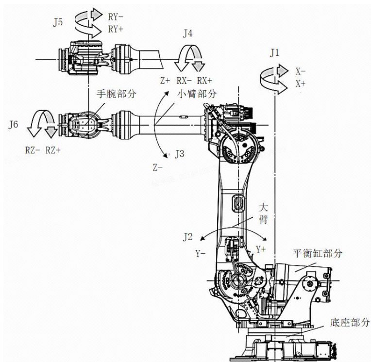
图 2-5 机械本体组成部分
