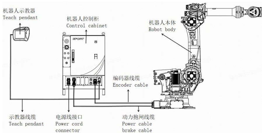
图 2-3 机器人系统构成
