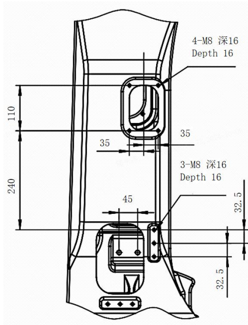
图 3-11 大臂上安装外部件尺寸图
