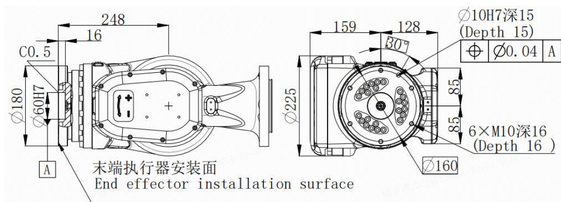
图 3-9 ER210-2700 V4 及 ER150-2700 末端负载安装法兰尺寸及末端负载安装尺寸
