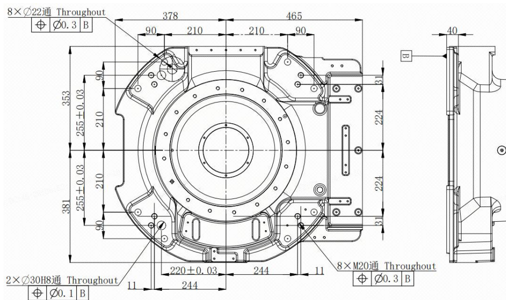
图 3-5 机器人底座尺寸
