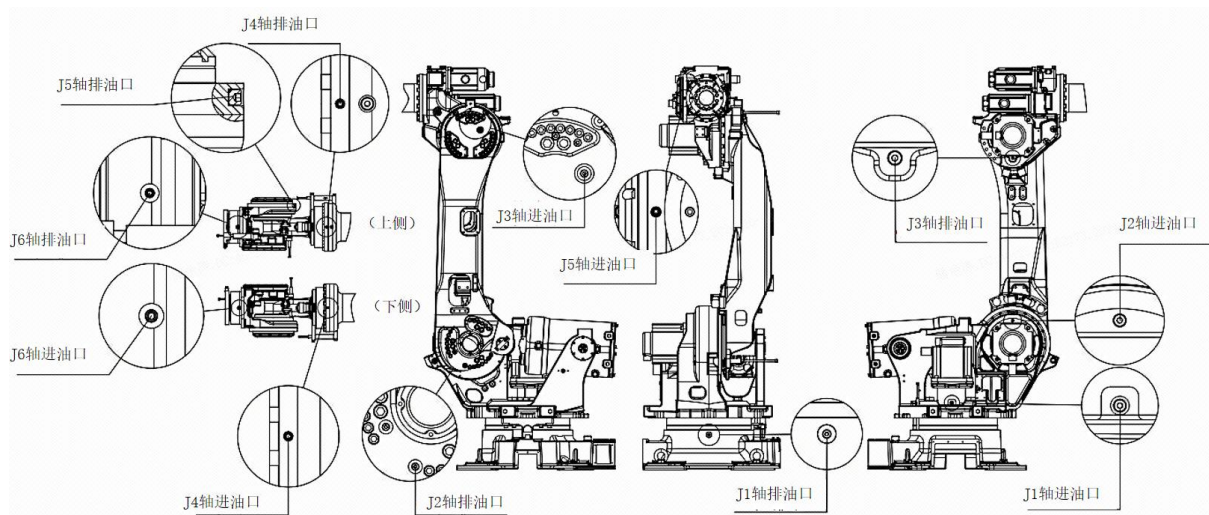
图 4-1 ER210-2700 V2 供脂口和排气口分布图
