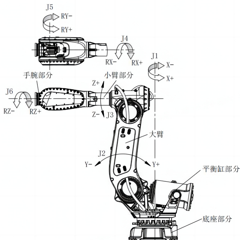
图 2-3 ER300 系列机械本体组成部分
