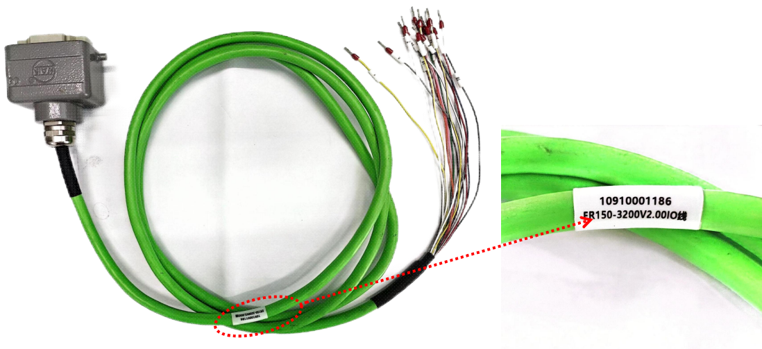
图 3-11 附送 IO 线示意图
