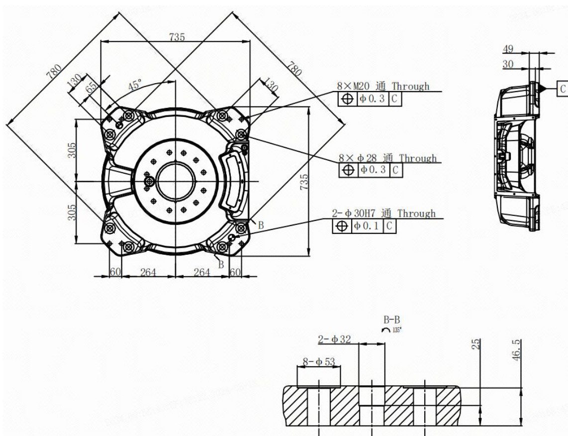
图 3-5 机器人底座尺寸
