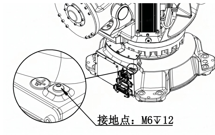
(c) 接地点示意图
