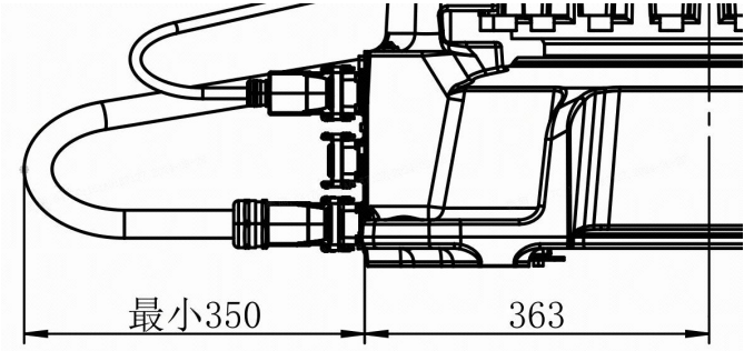
图 3-6 底座线缆后侧出线最小弯折尺寸
