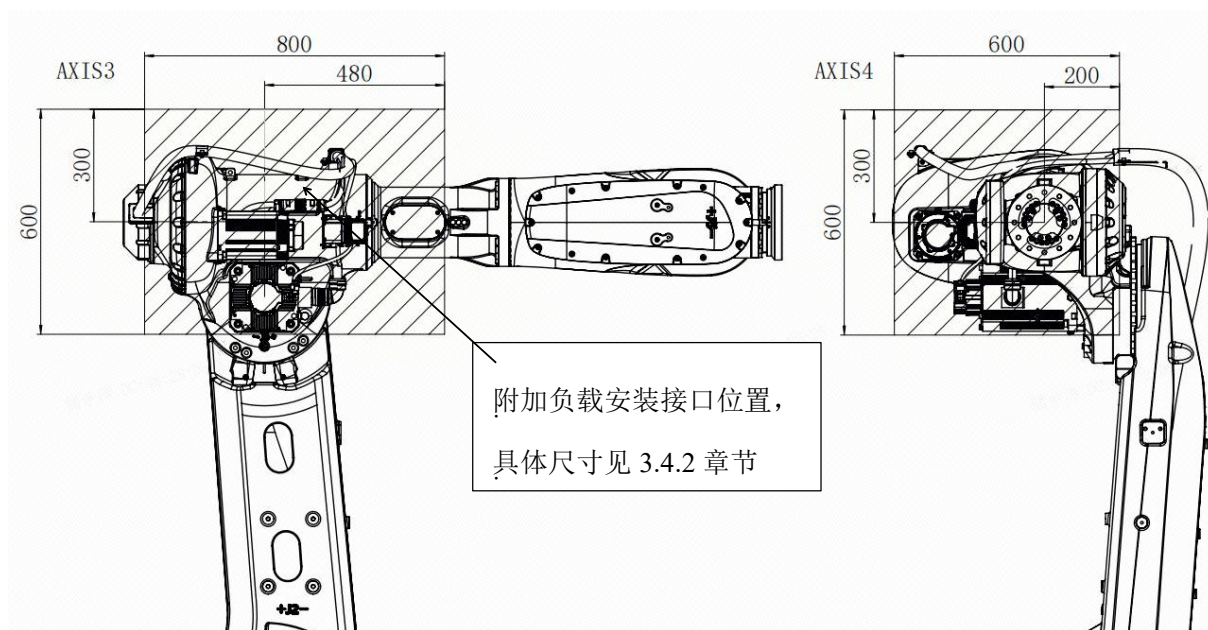
图 2-8 ER300 系列上臂附加负载质心范围图
