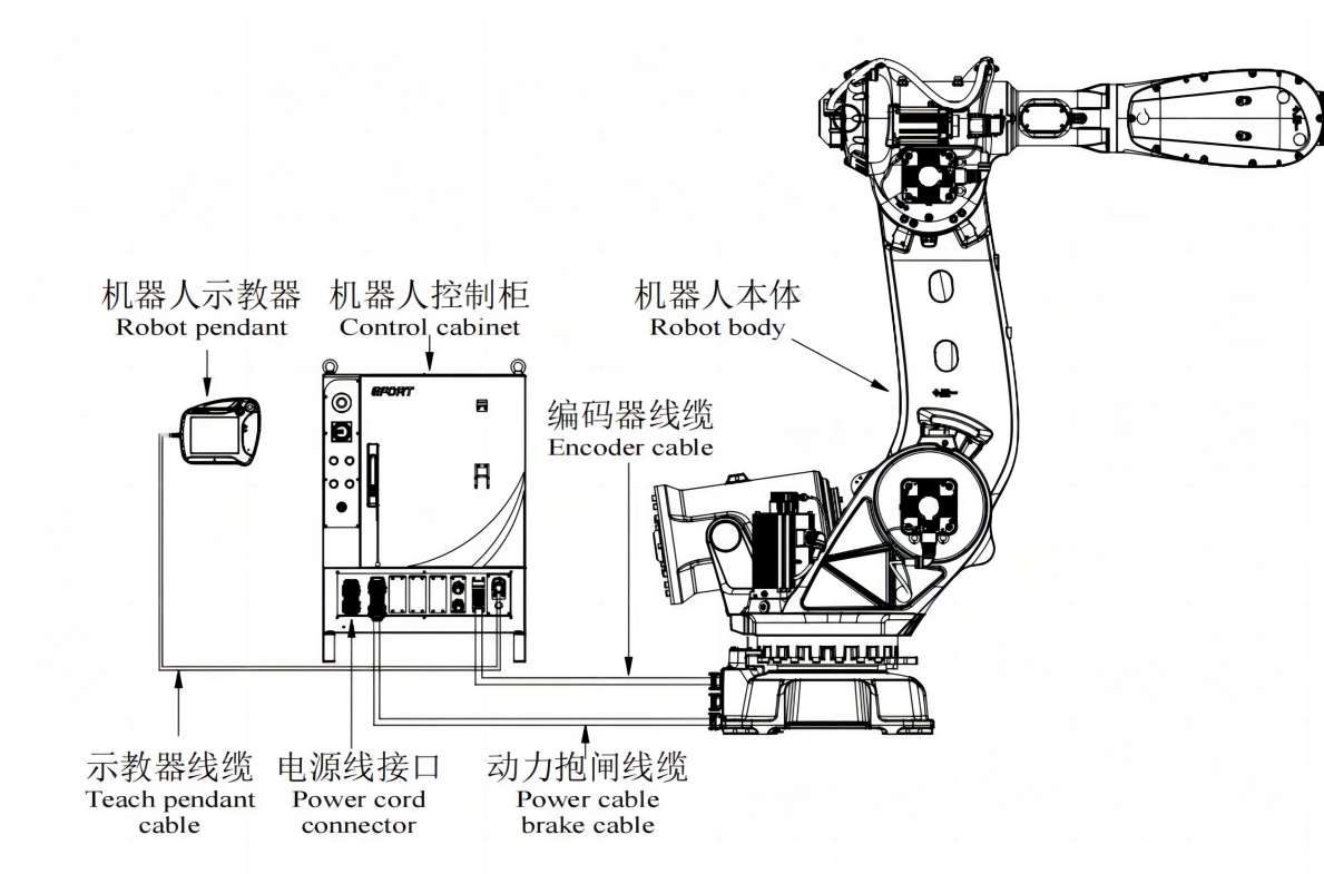
图 2-1 工业机器人系统构成
