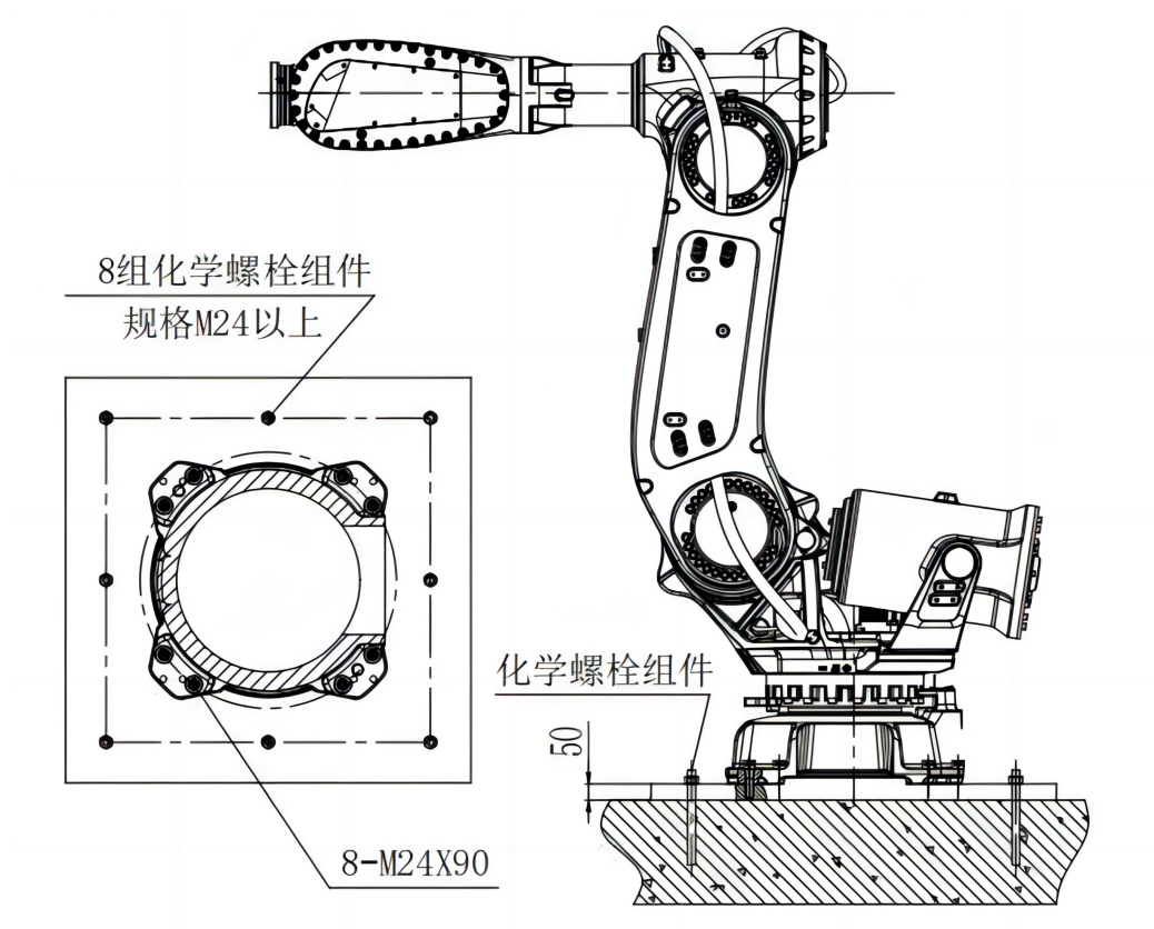
图 3-7 机器人安装举例
