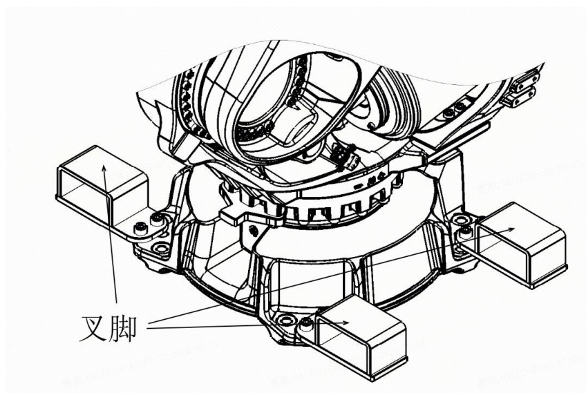
图 3-2 叉脚安装示意图
