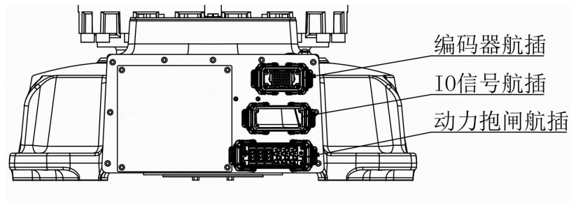
图 3-13 底座部分信号线接口
