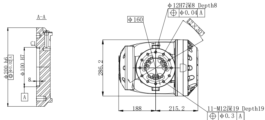
末端法兰安装图 (End flange mounting size)
