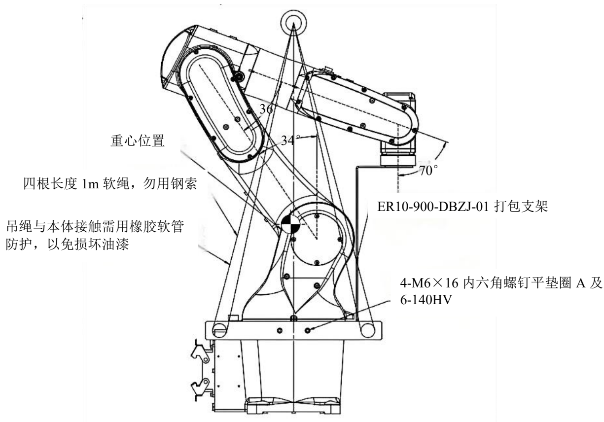
图 3-1 吊装搬运示意图
