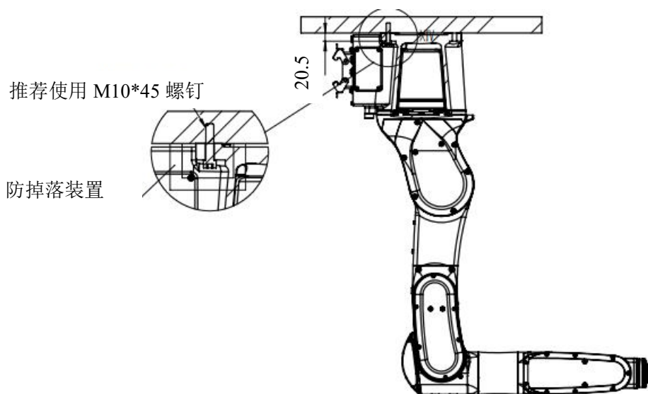
图 3-4 倒挂安装
