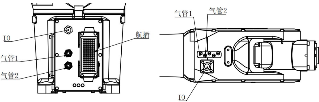
图 3-9 IO 气管位置示意图
