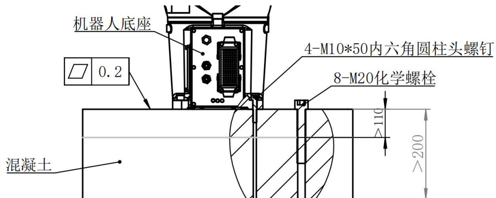
图 3-3 机器人安装举例
