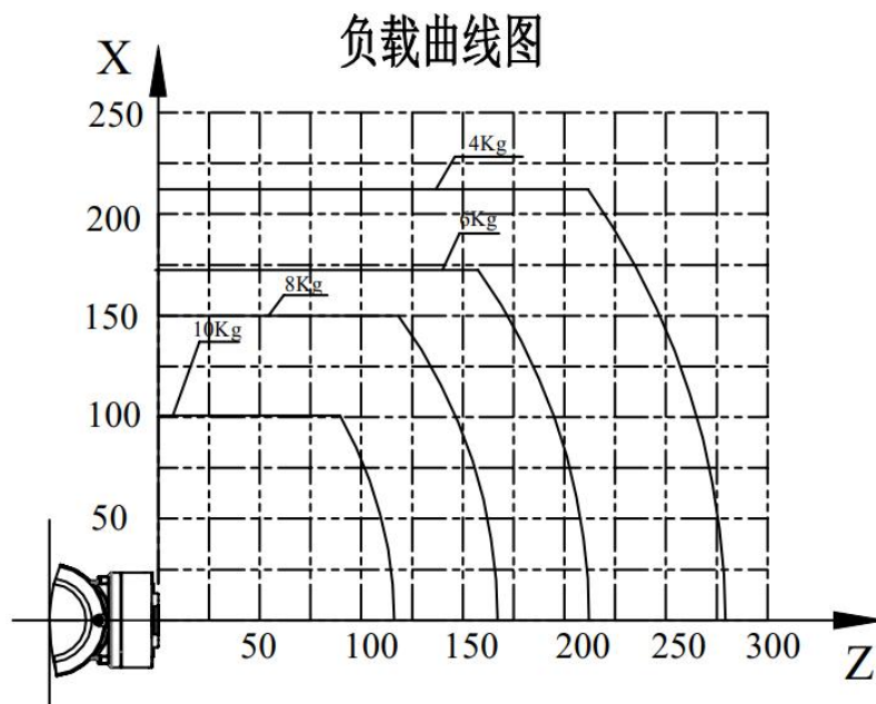
图 2-6 ER10-900 手腕轴转矩图
