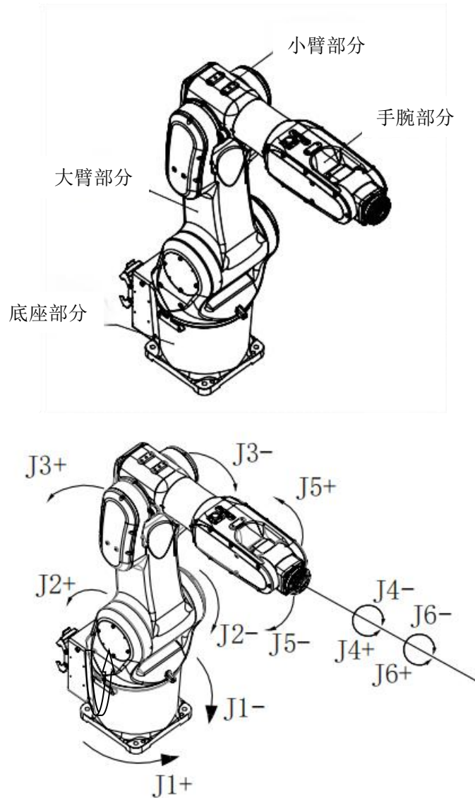
图 2-3 ER10-900 机械本体组成部分
