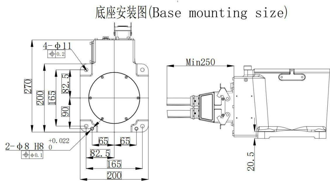
图 3-2 机器人底座尺寸
