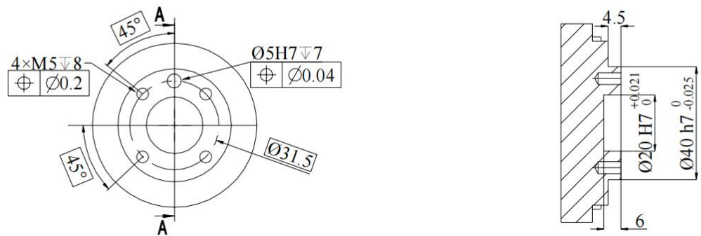
图 3-6 末端负载安装法兰尺寸
