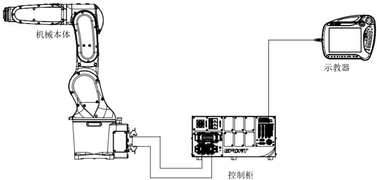
图 2-1 工业机器人系统构成
