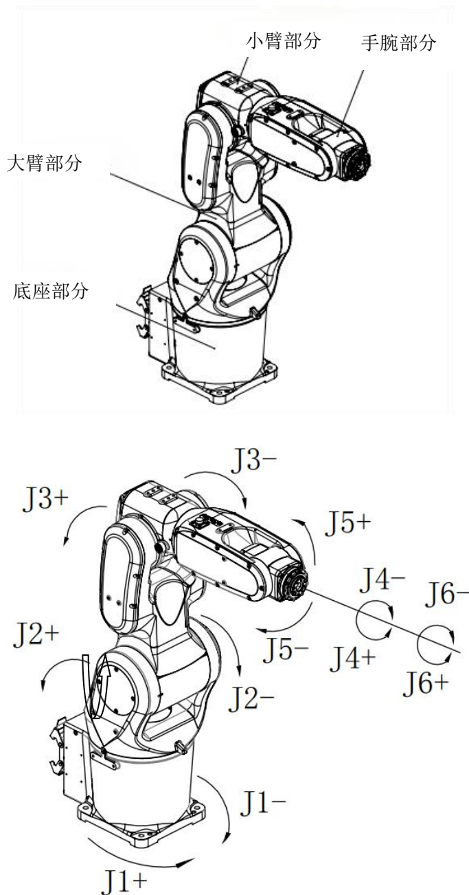
图 2-3 ER10-700 机械本体组成部分
