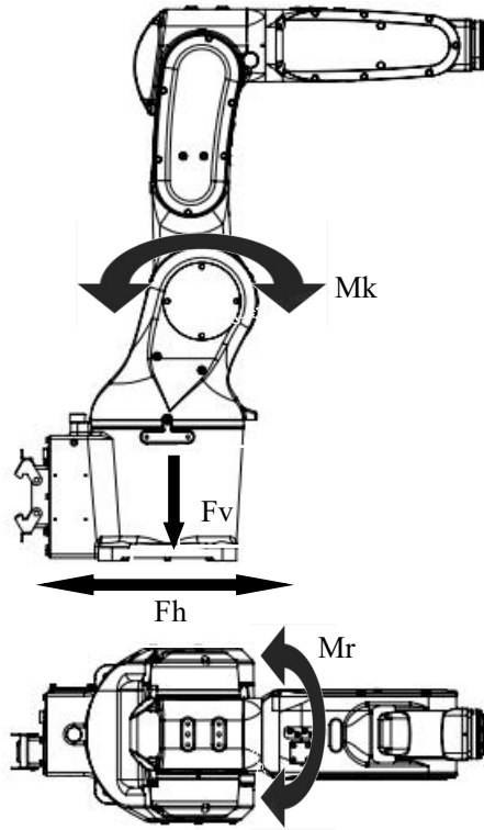
图 3-5 机器人受力图
