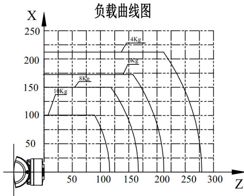
图 2-6 ER10-700 手腕轴转矩图
