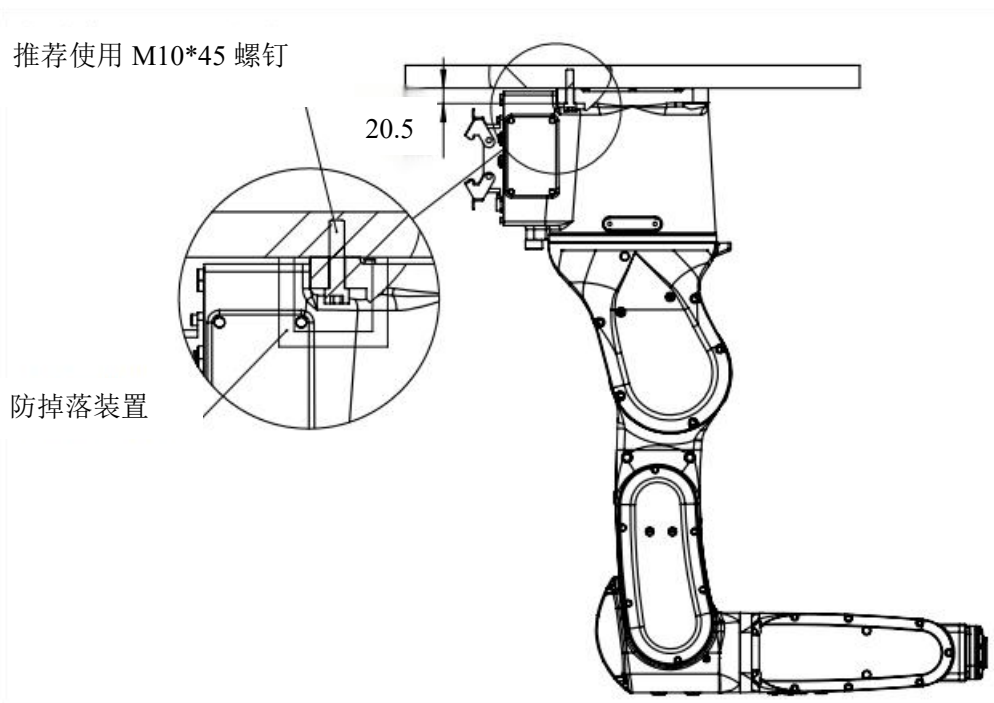
图 3-4 倒挂安装
