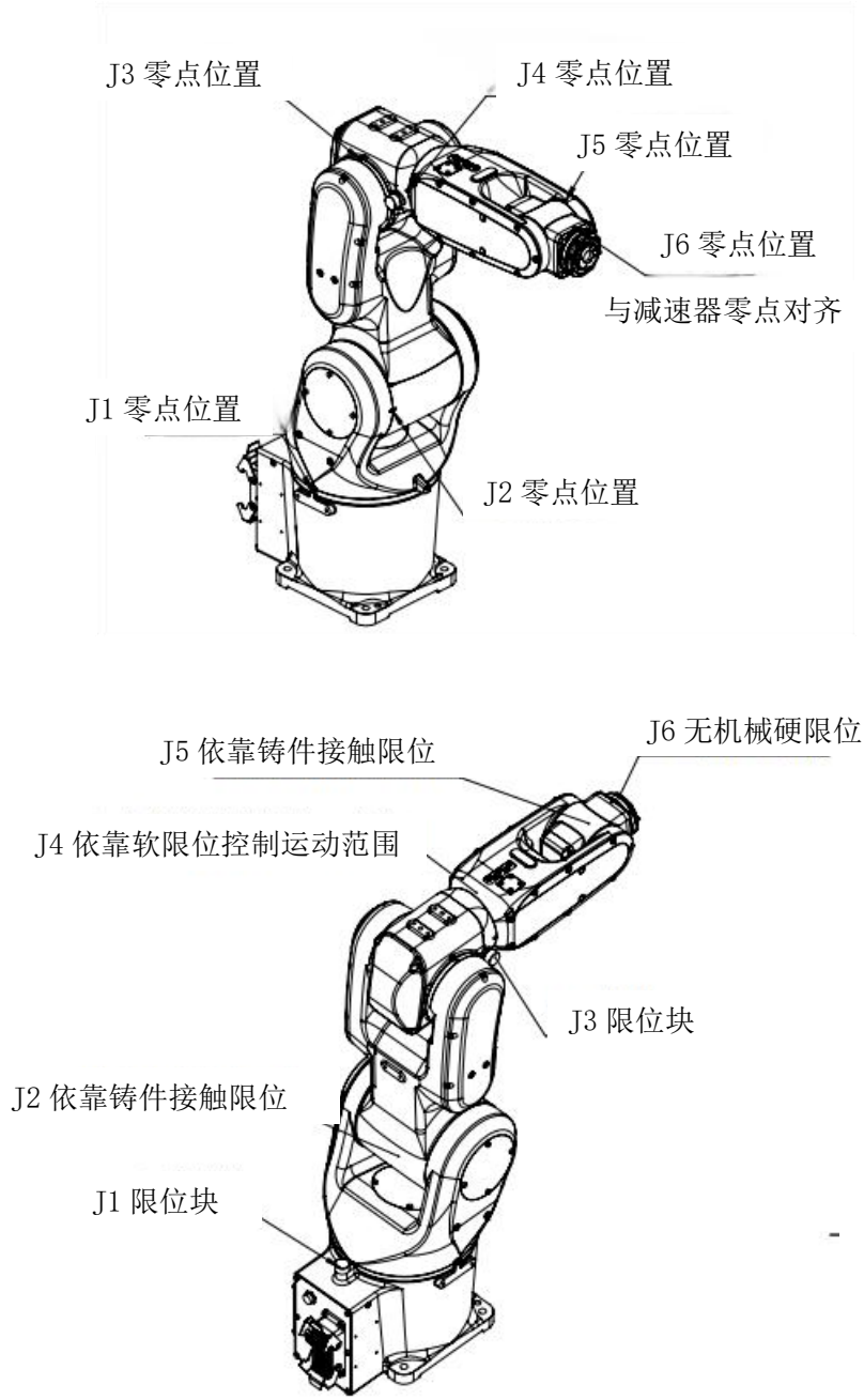
图 2-4 机械硬限位位置及零标位置
