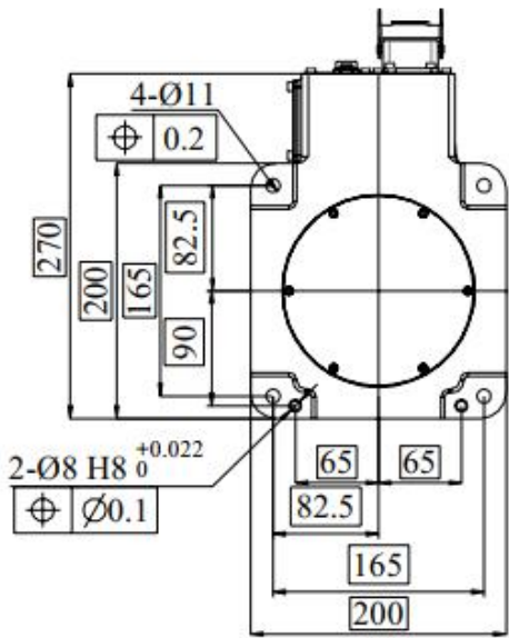
图 3-2 机器人底座尺寸
