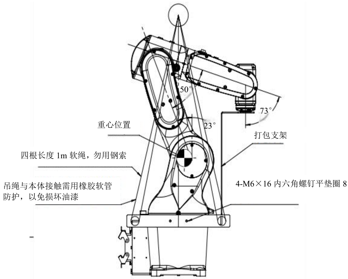
图 3-1 吊装搬运示意图
