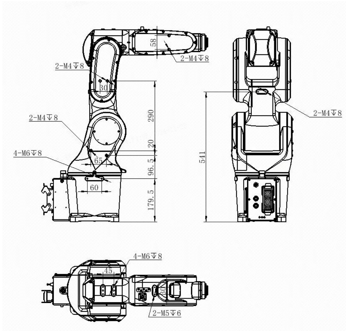
图 3-7 外围安装尺寸图
