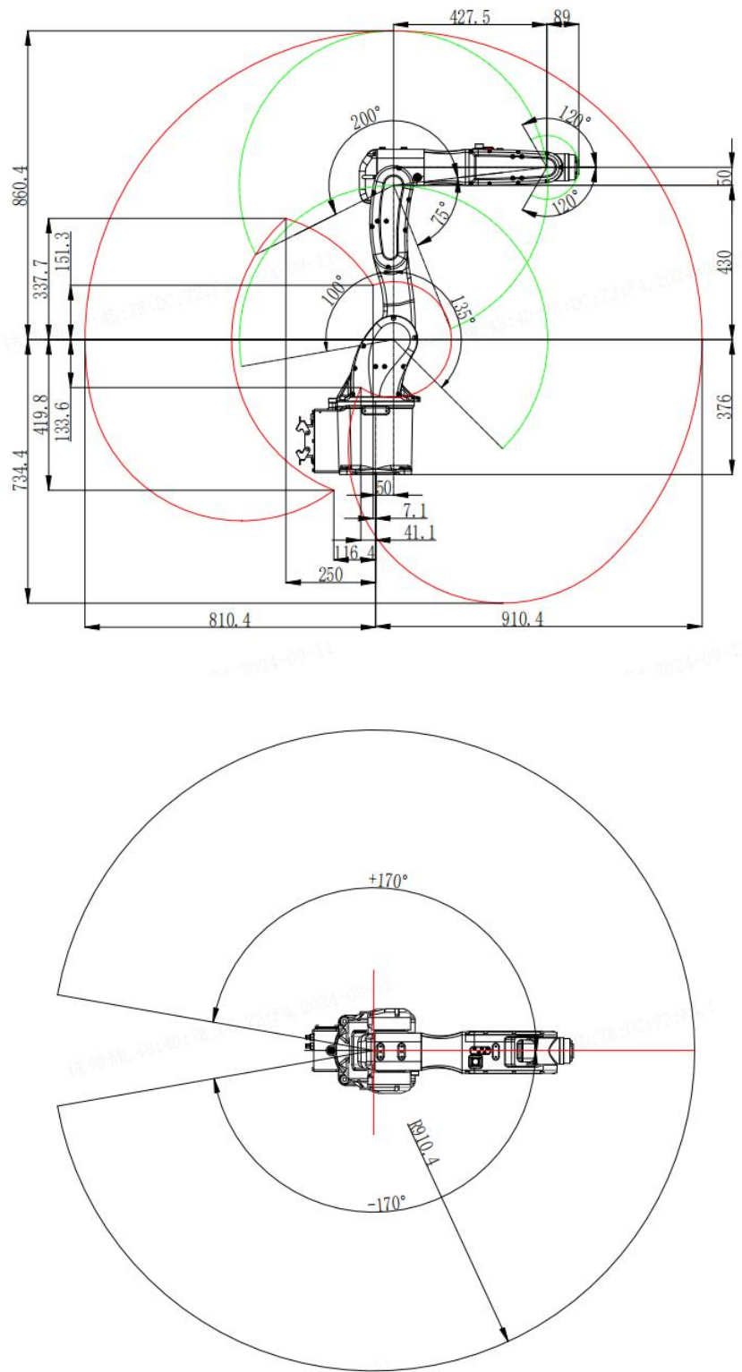
图 2-5 机器人工作空间图
