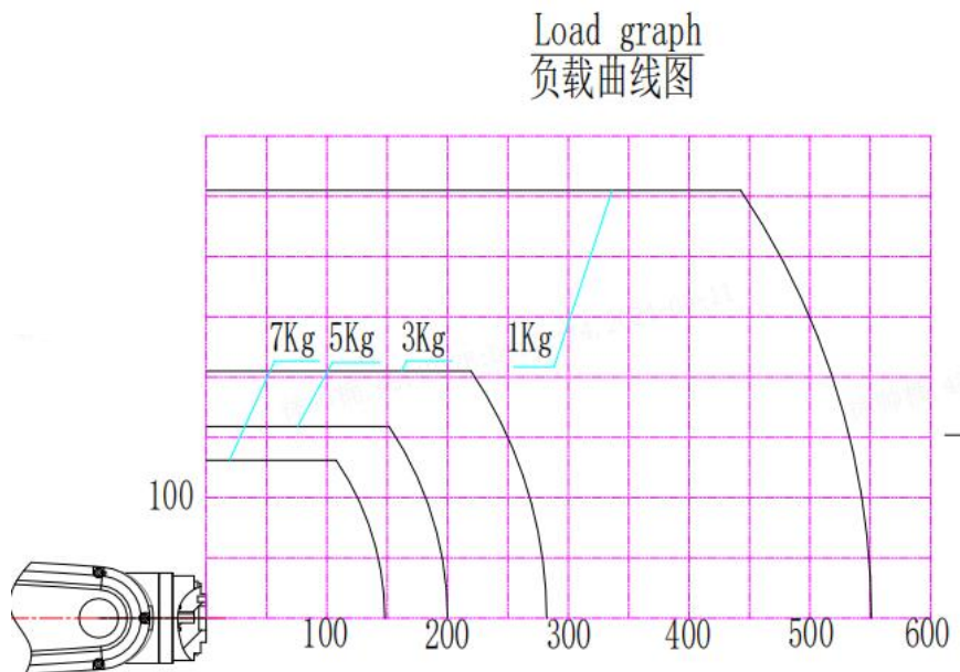
图 2-6 ER7-900 手腕轴转矩图
