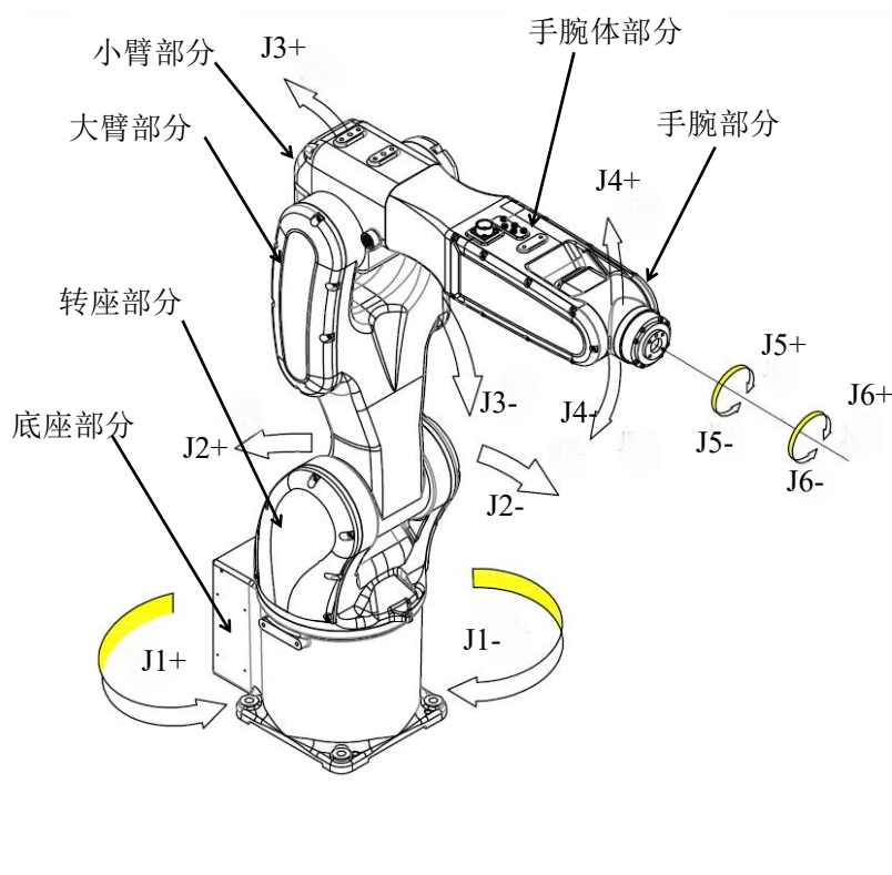
图 2-3 ER7-900 机械本体组成部分
