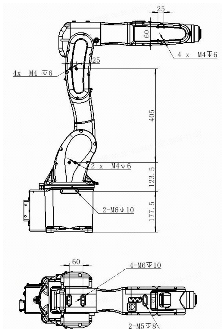
图 3-6 安装外部件尺寸图
