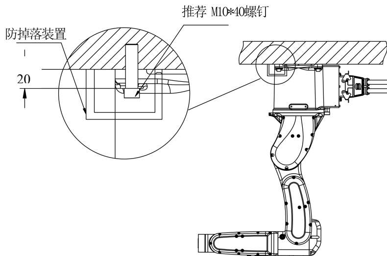
图 3-4 倒挂安装
