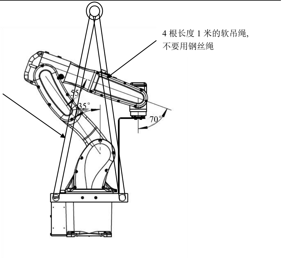
图 3-1 吊装搬运示意图
