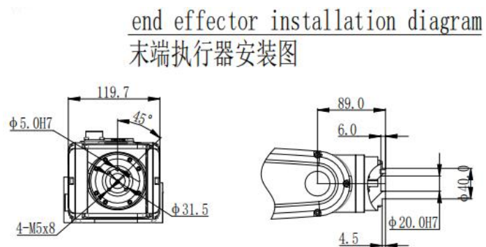
图 3-5 末端负载安装法兰尺寸
