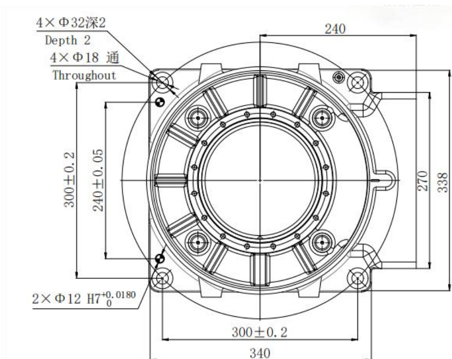
图 3-4 机器人底座尺寸
