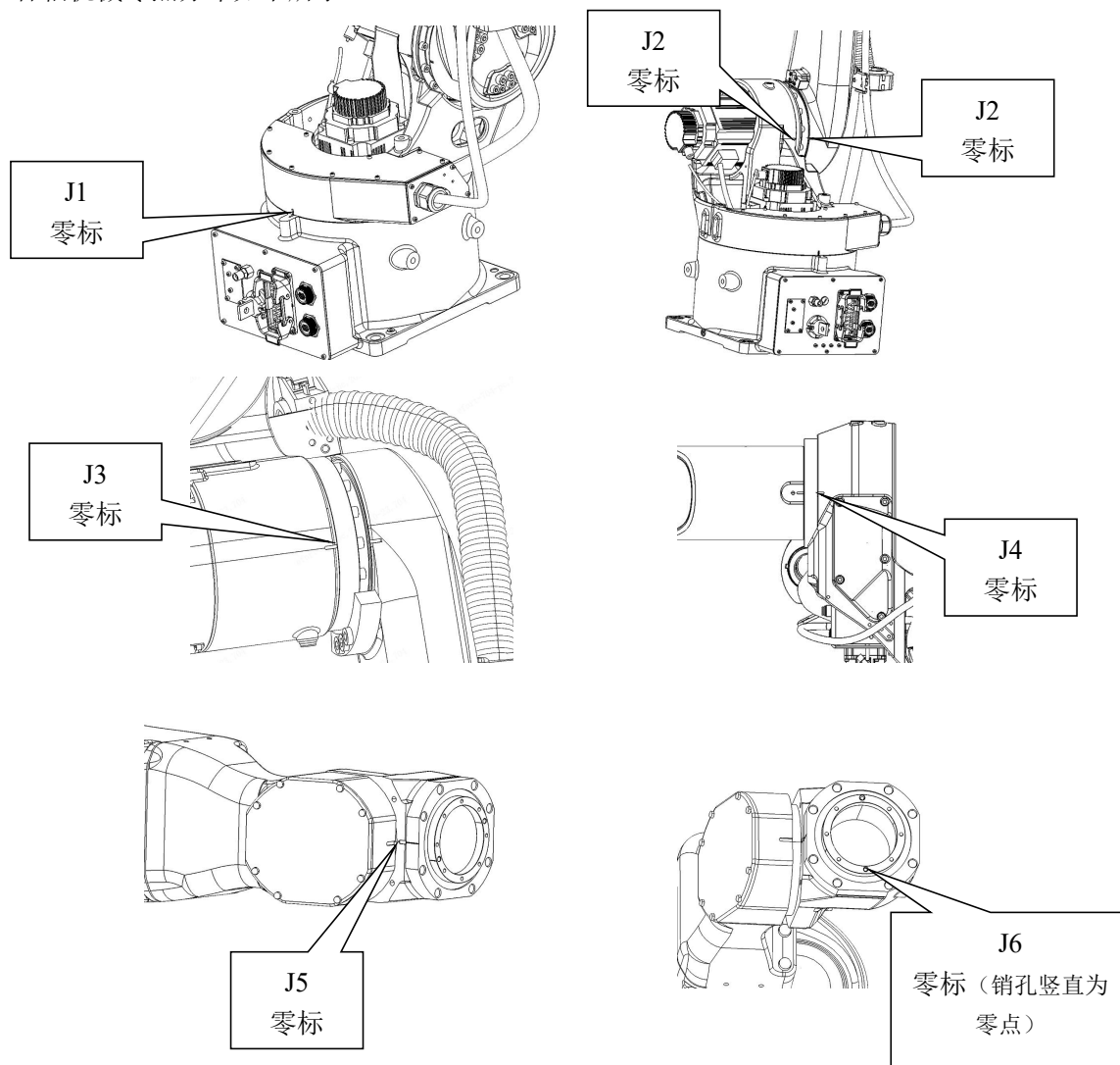
图 4-3 机器人零点位置图
