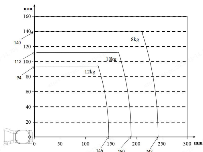
图 2-6 ARC12-1400 手腕轴转矩图
