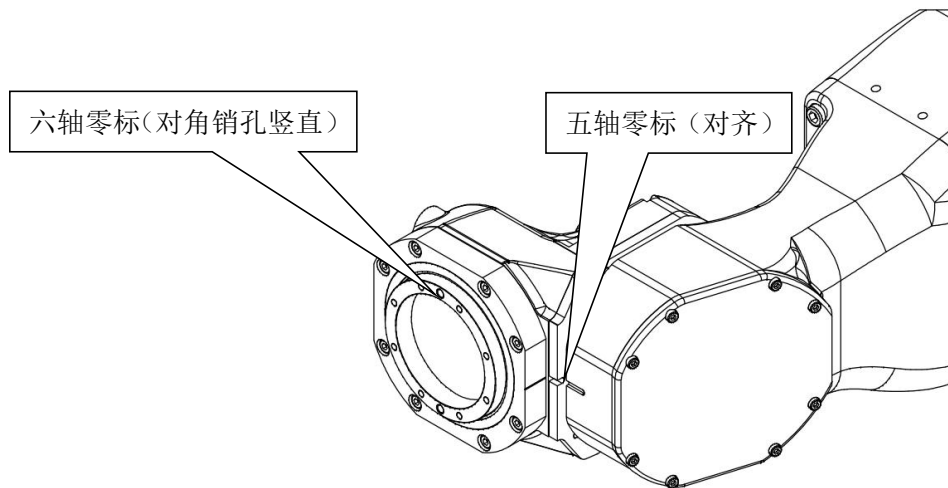
图 2-4 机械硬限位位置及零标位置
