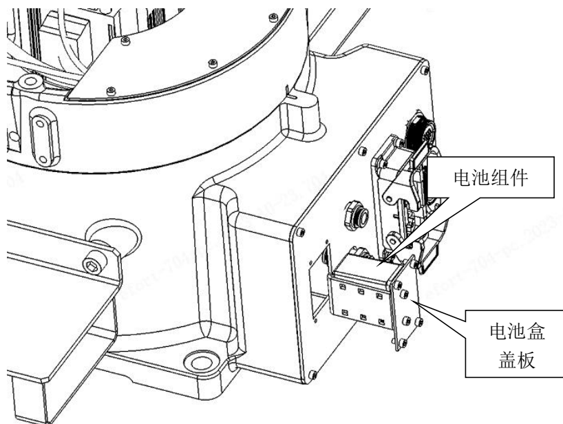
图 4-4 机器人电池组位置图
