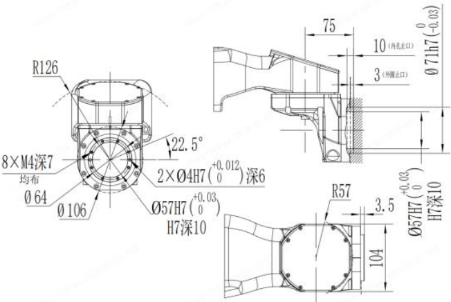
图 3-9 末端负载安装法兰尺寸
