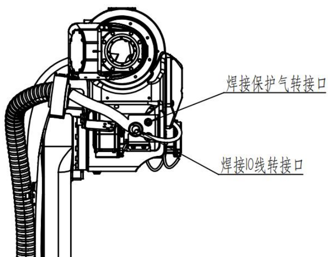
图 3-12 电机座部分气路及信号线接口
