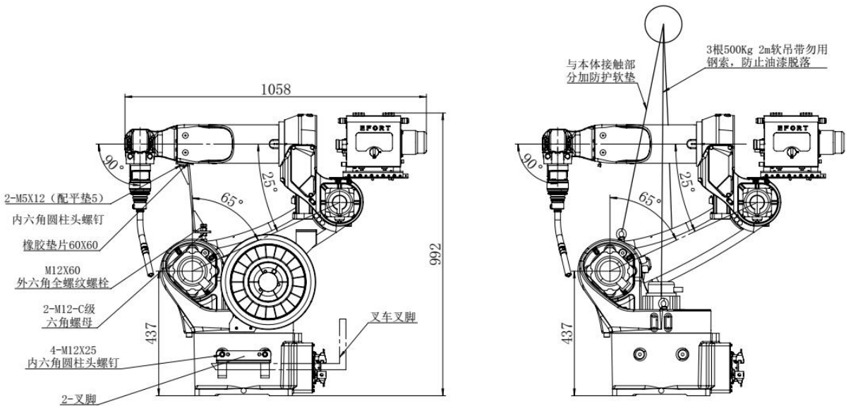
图 3-3 转运示意图
