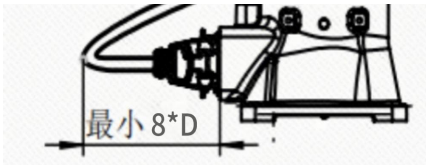
图 3-5 底座线缆后侧出线最小弯折尺寸
