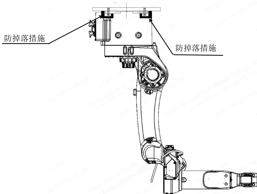
图 3-7 机器人倒装案例
