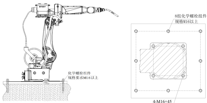
图 3-6 机器人安装举例
