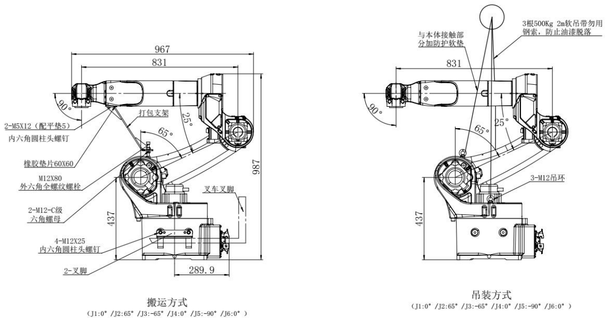
图 3-3 转运示意图
