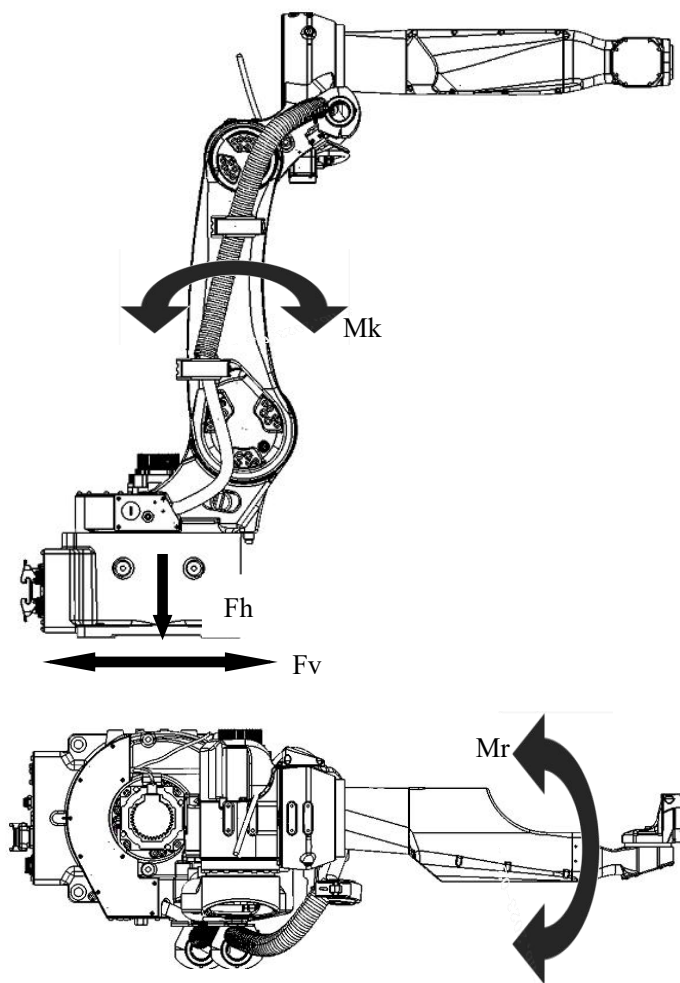
图 3-8 机器人受力图
