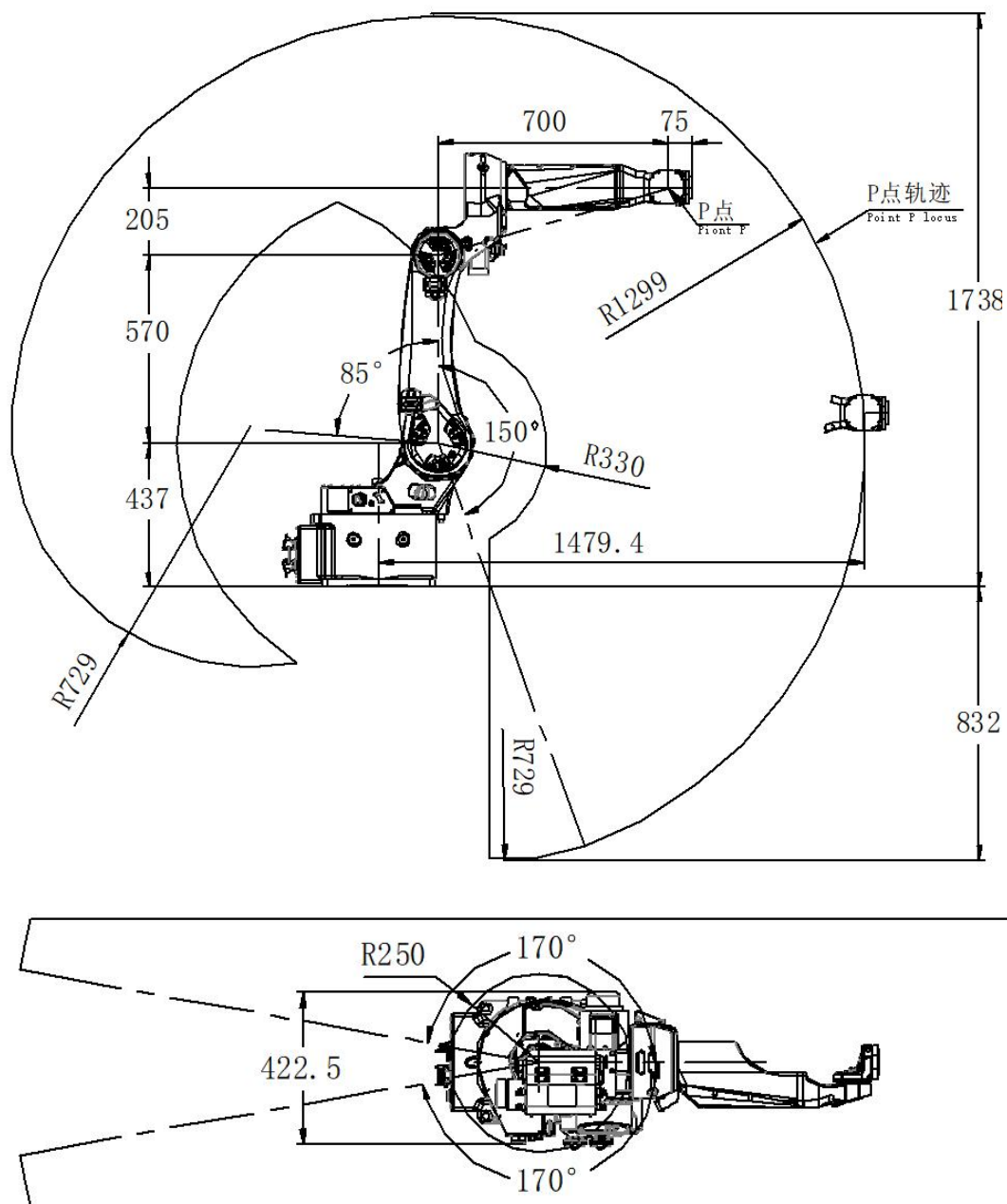
图 2-5 机器人工作空间图
