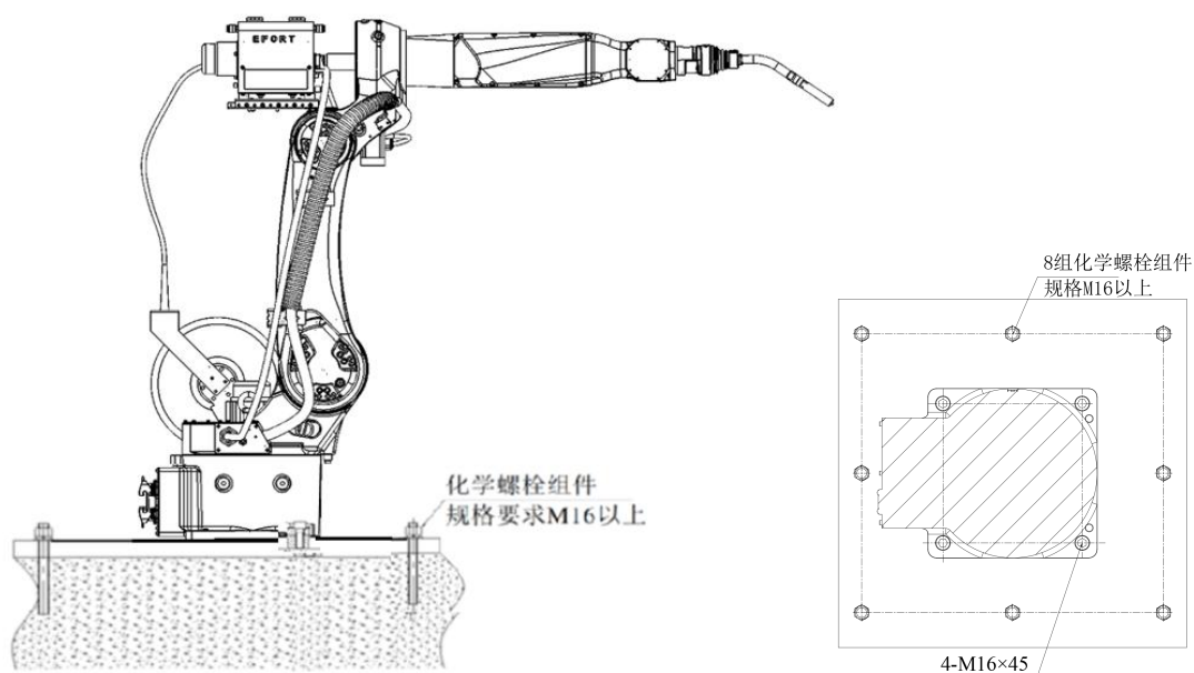
图 3-6 机器人安装举例
