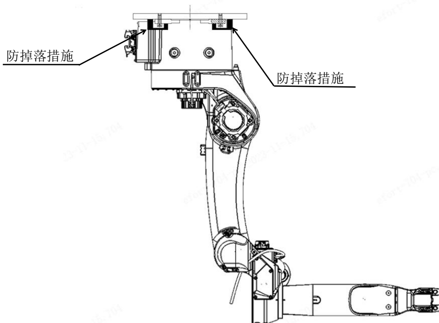
图 3-7 机器人倒装案例
