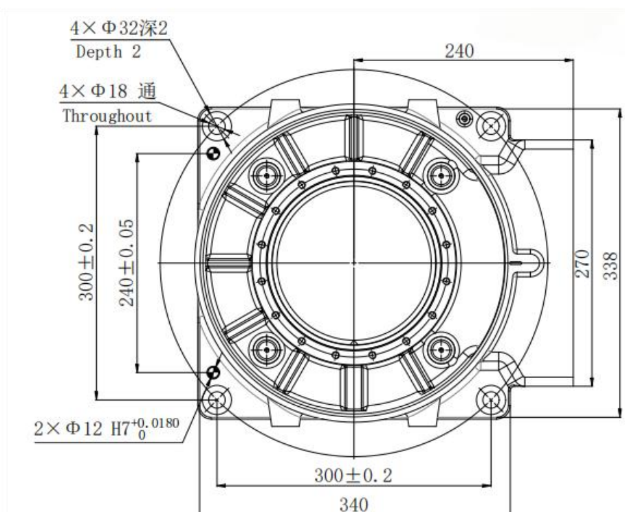
图 3-4 机器人底座尺寸
