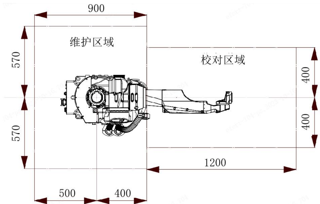
图 4-2 维护及使用区域
