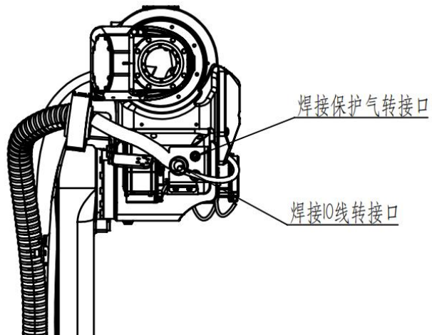
图 3-13 电机座部分气路及信号线接口
