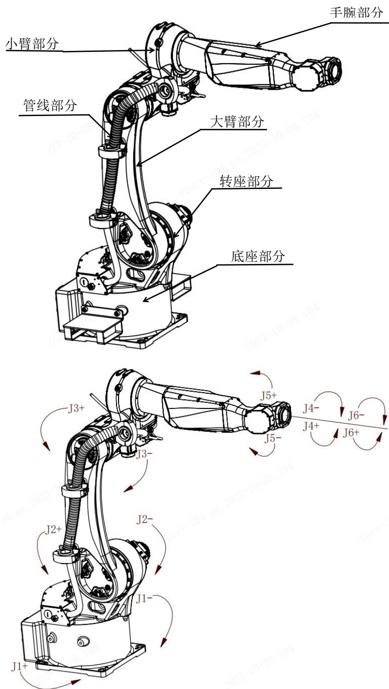
图 2-3 ARC10-1600 机械本体组成部分
