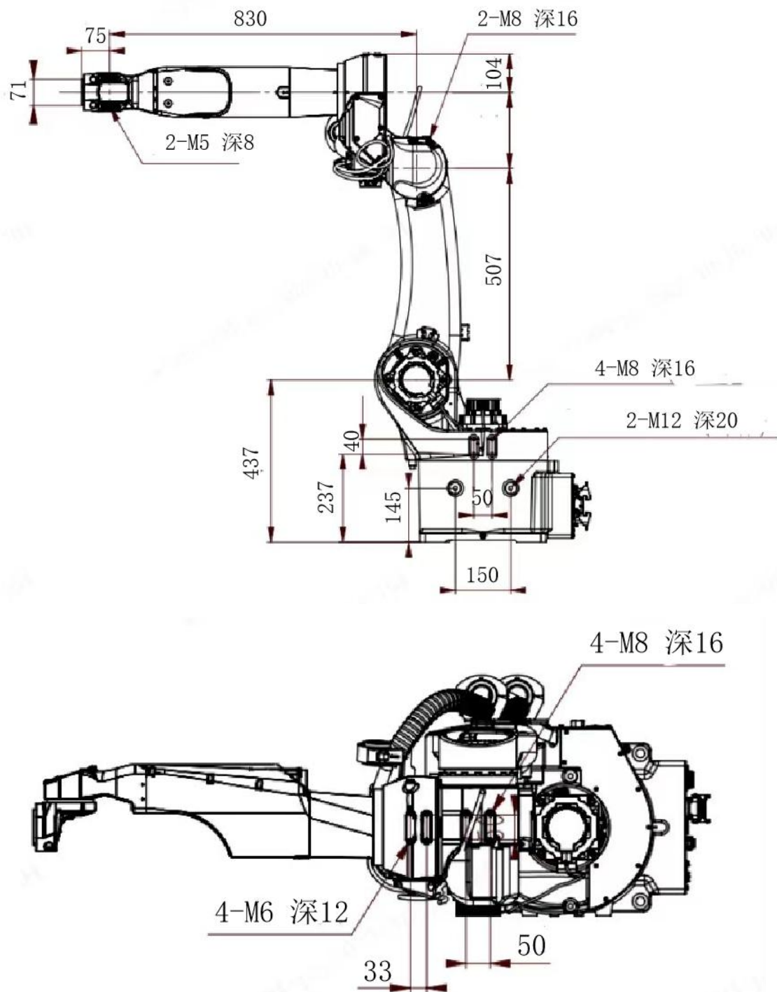
图 3-10 外围安装尺寸图
