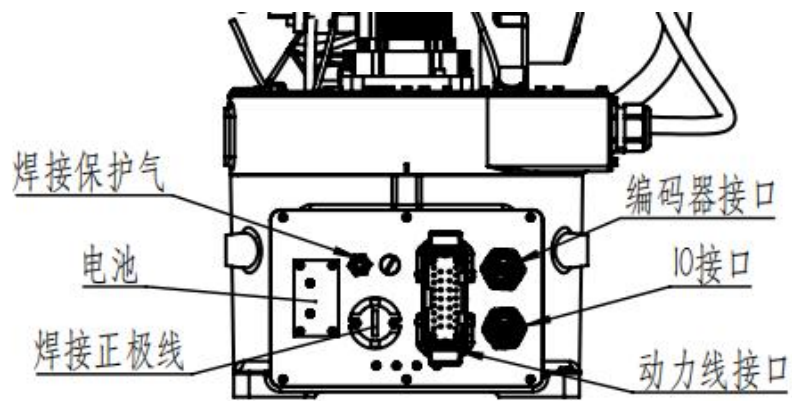
图 3-12 底座部分气路及信号线接口
