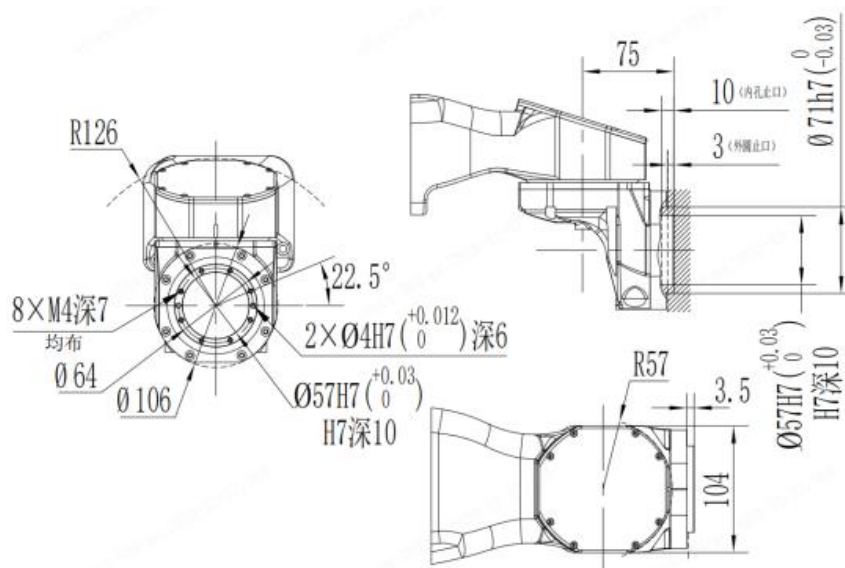
图 3-9 末端负载安装法兰尺寸
