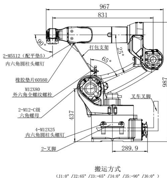
图 3-1 打包固定支架安装示意图
