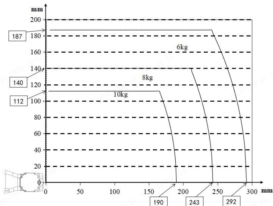
图 2-6 ARC10-1600 手腕轴转矩图
