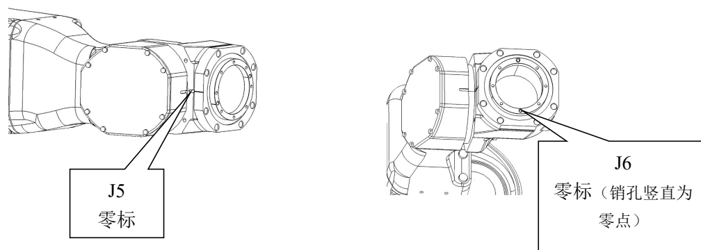
图 4-3 机器人零点位置图
