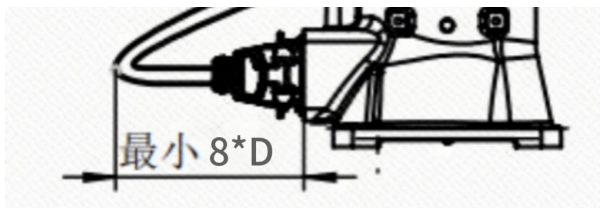
图 3-5 底座线缆后侧出线最小弯折尺寸
