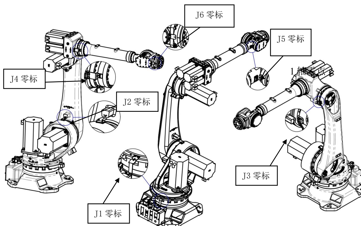
图 4-3 机器人零点位置图
