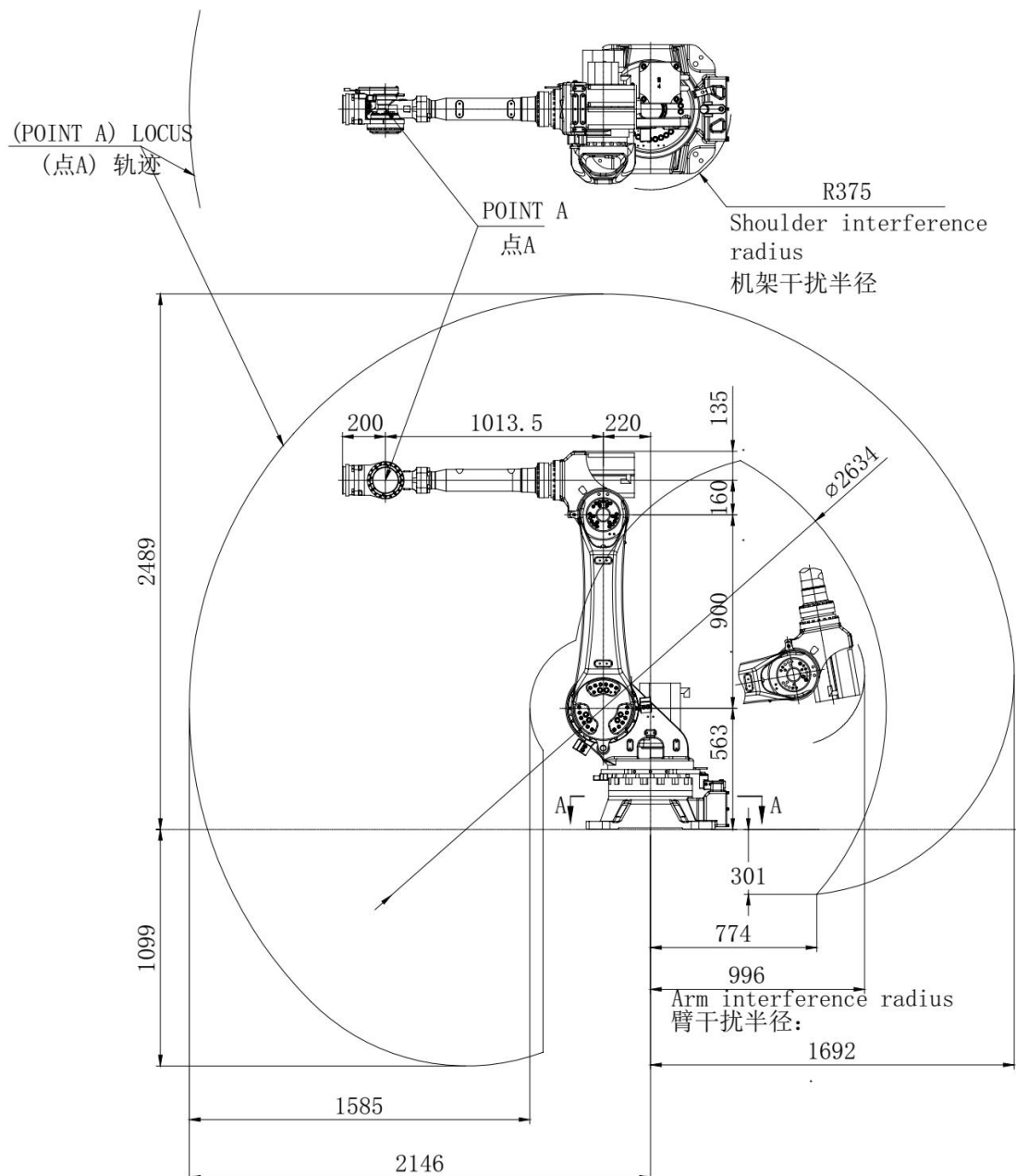
图 2-8 机器人工作空间图
