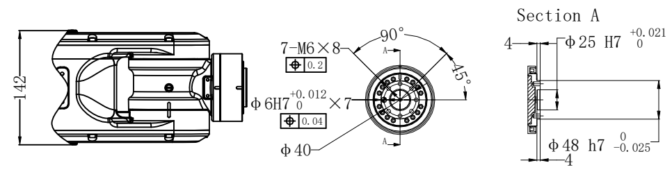
末端法兰安装图 (End flange mounting size)
