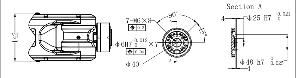
末端法兰安装图 (End flange mounting size)
