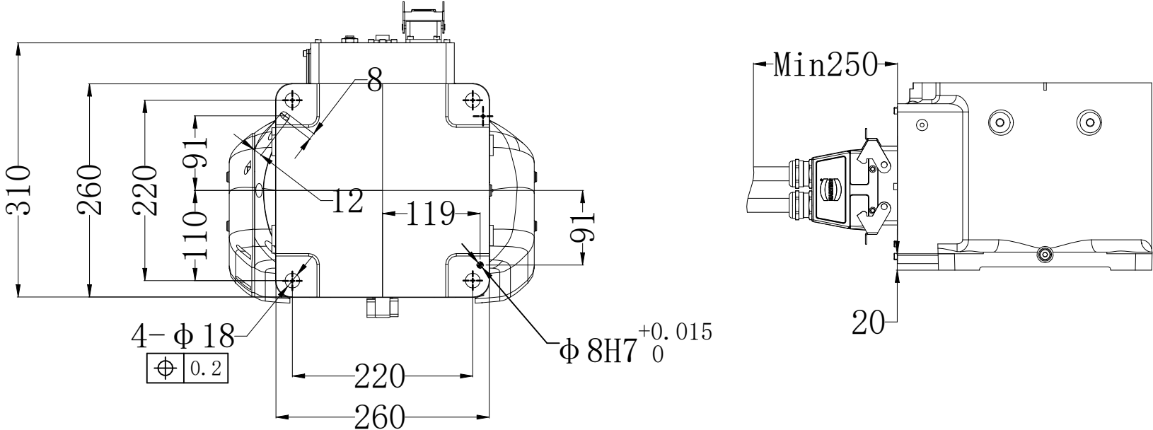
末端法兰安装图 (End flange mounting size)
