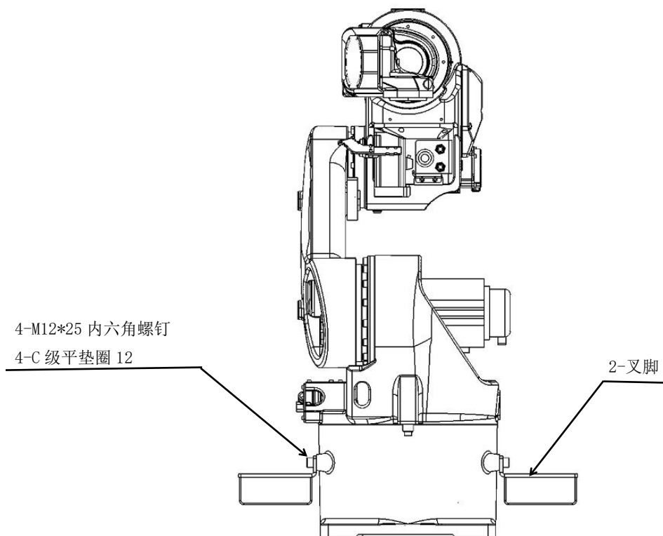
图 3-2 叉脚安装示意图
