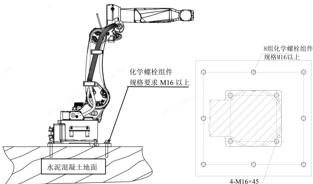
图 3-5 机器人安装举例
