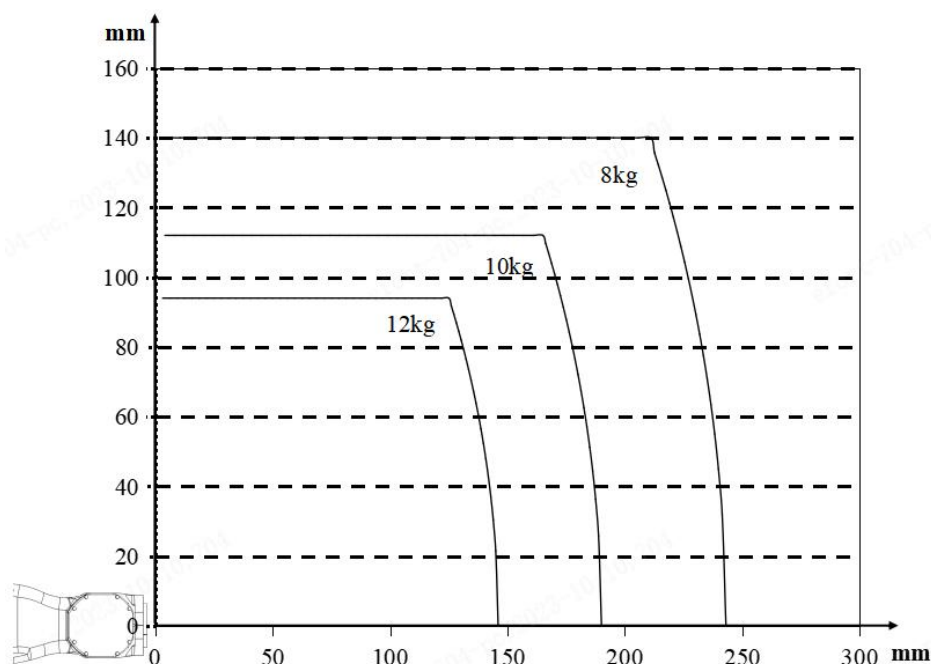
图 2-6 ER12H-1600 手腕轴转矩图
