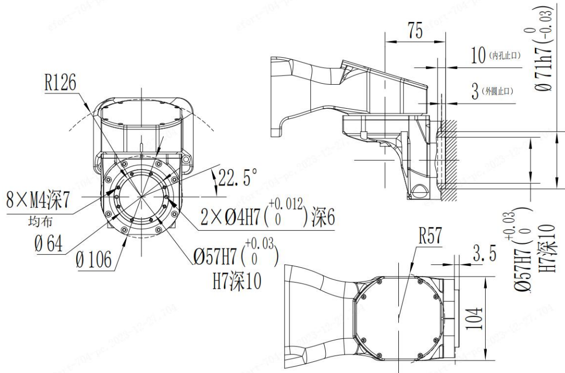
图 3-7 末端负载安装法兰尺寸
