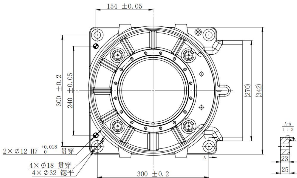
图 3-4 机器人底座尺寸
