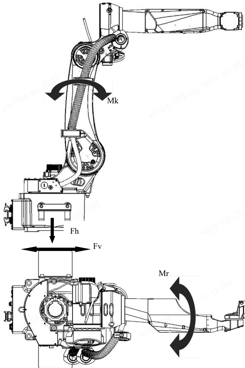
图 3-6 机器人受力图
