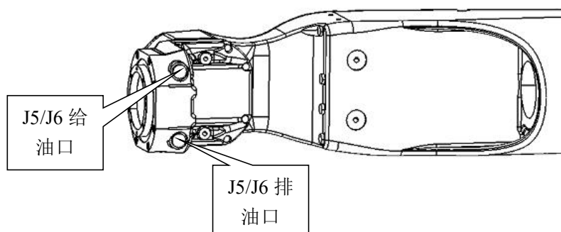
图 4-1 机器人进油口和出油口分布图
