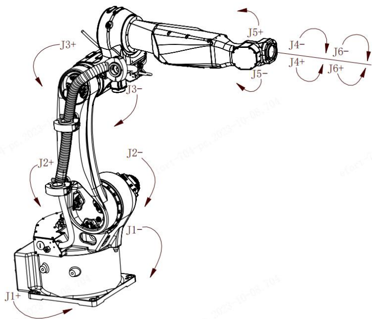
图 2-3 ER12H-1600 机械本体组成部分
