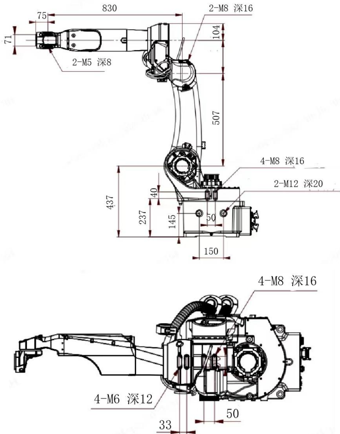
图 3-8 外围安装尺寸图
