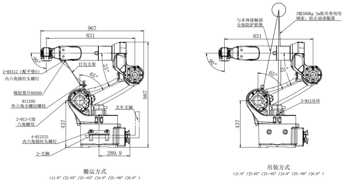
图 3-3 转运示意图（左侧叉车转运、右侧行车吊装）
