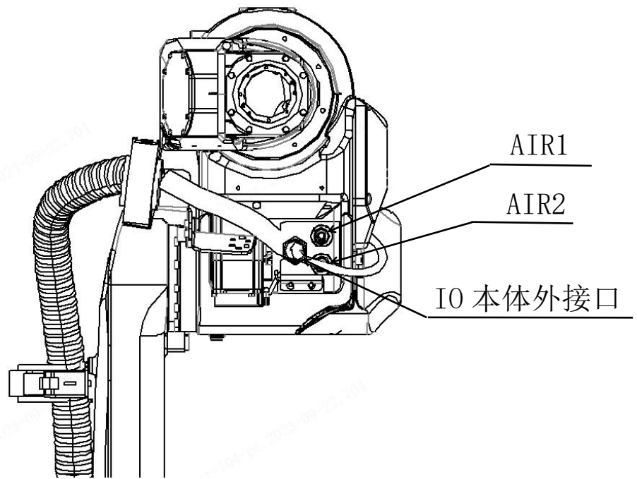
图 3-11 电机座部分气路及信号线接口
