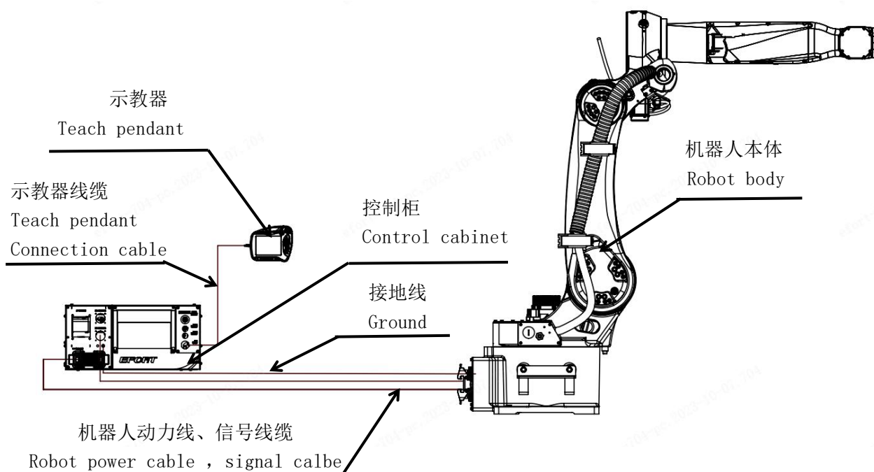
图 2-1 工业机器人系统构成
