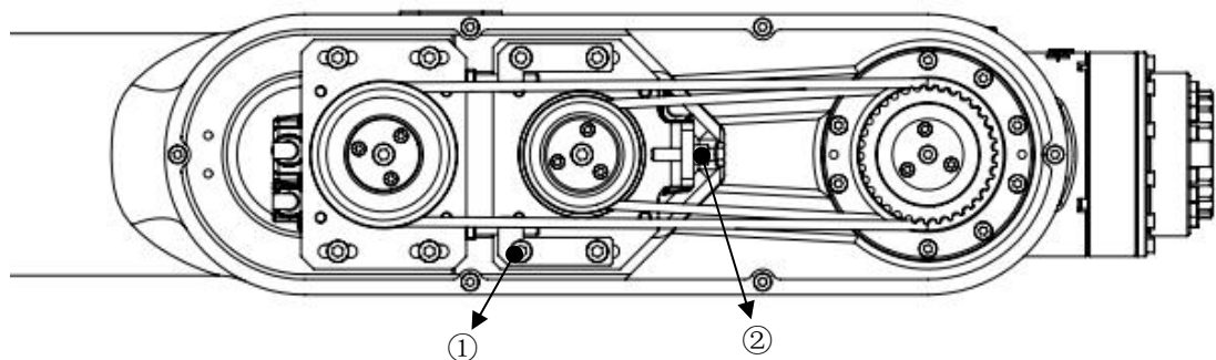
注：①固定螺钉，4 个 M5×20；②调距螺钉，1 个 M5×25
