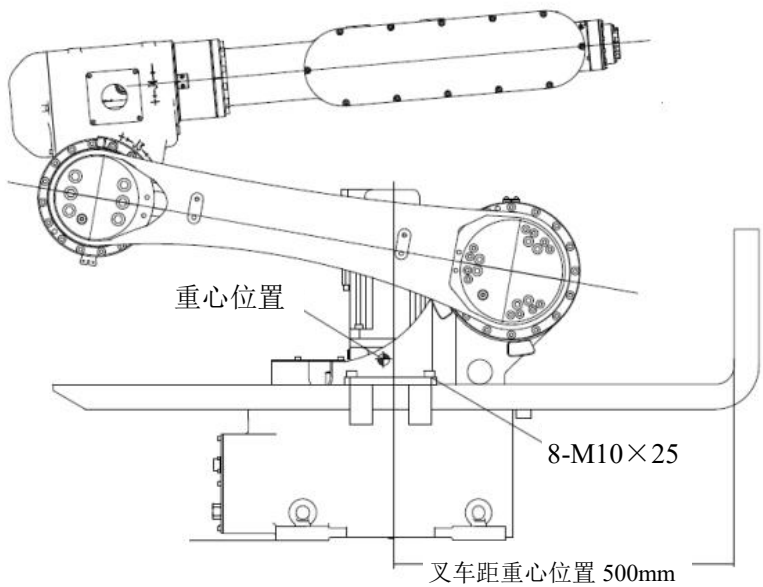
图 3-4 叉车搬运示意图
