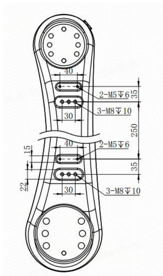
图 3-10 大臂上安装外部件尺寸图
