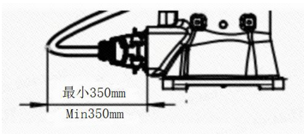
图 3-6 底座线缆后侧出线最小弯折尺寸
