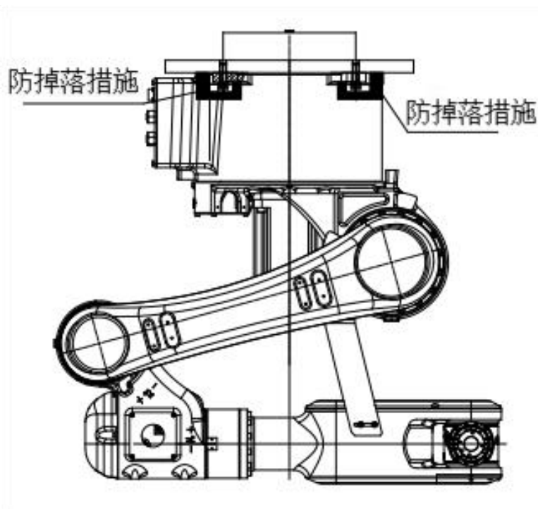
图 3-8 倒挂安装
