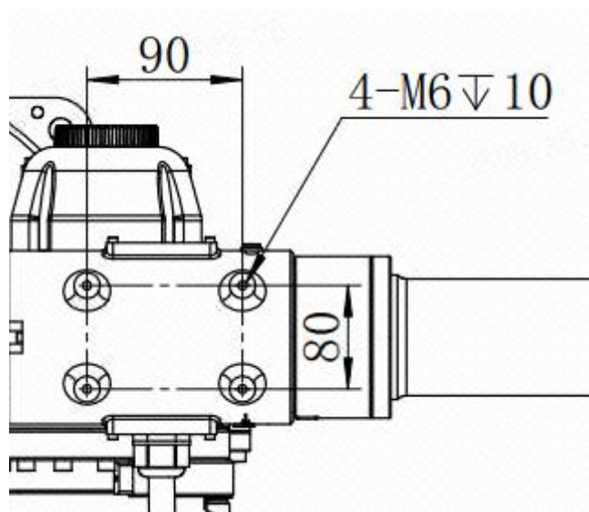
图 3-11 电机座上安装外部件尺寸图
