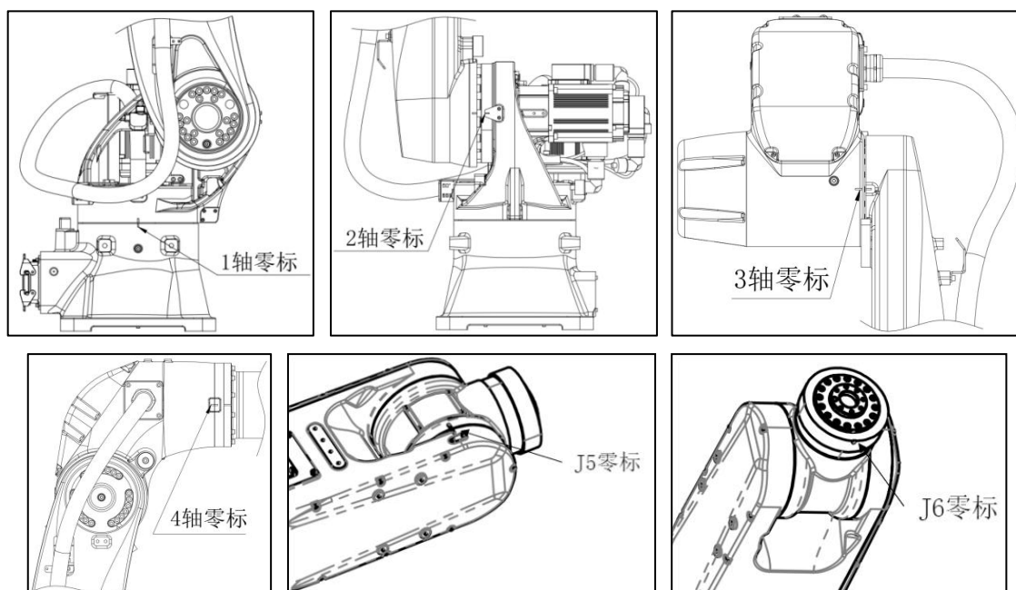
图 4-4 机器人零点位置图
