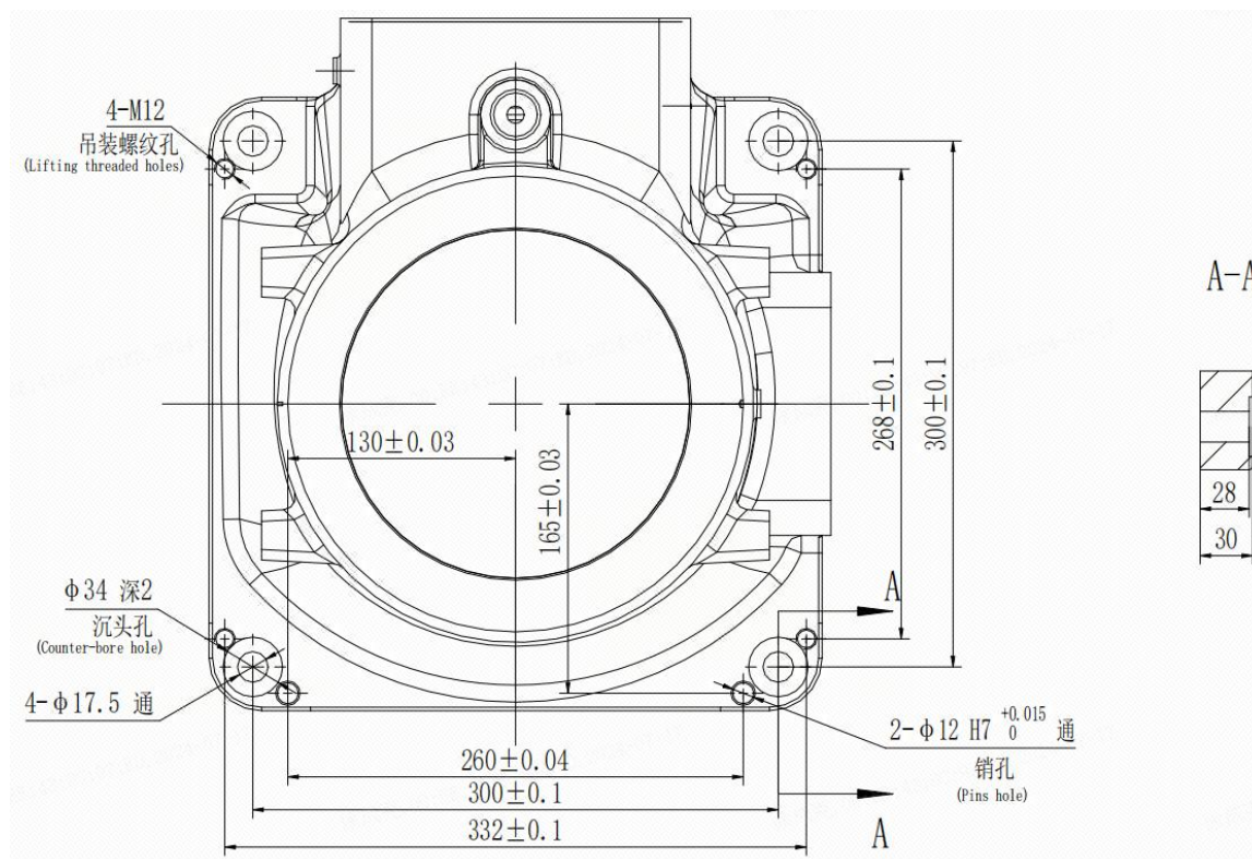
图 3-5 机器人底座尺寸
