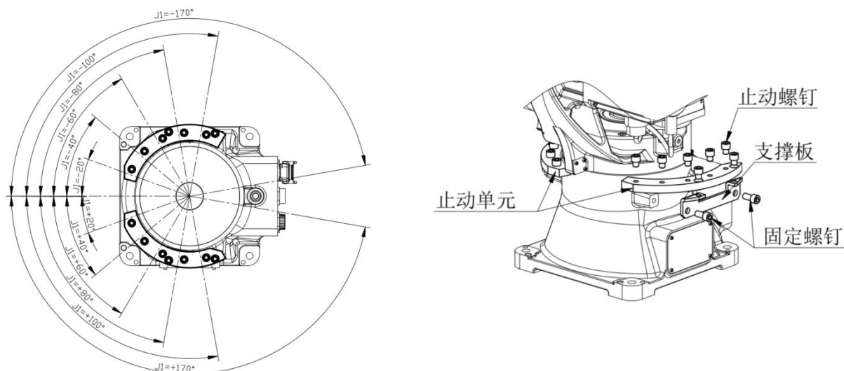
图 2-5 J1 轴可调限位图
