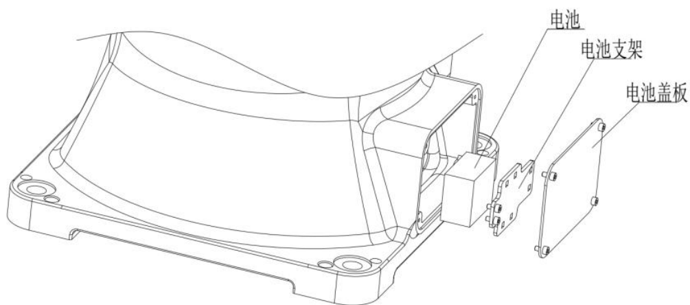
图 4-5 机器人电池组位置图
