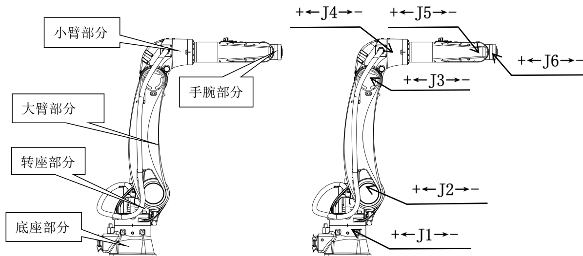
图 2-3 ER35-1800 机械本体组成部分
