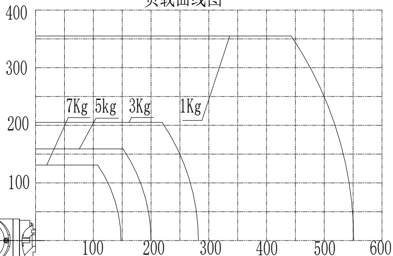
Load graph 负载曲线图
