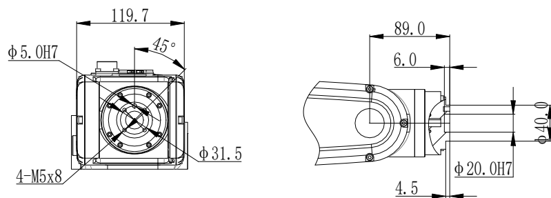
末端执行器安装图
