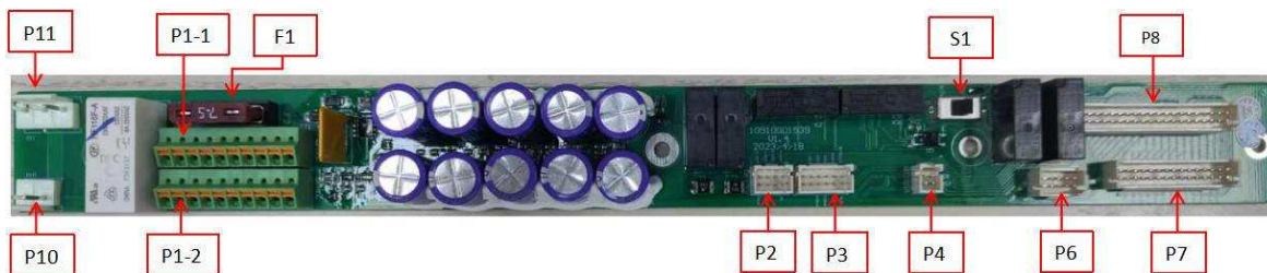
图 4.4.6 电源分配板接口分布说明
