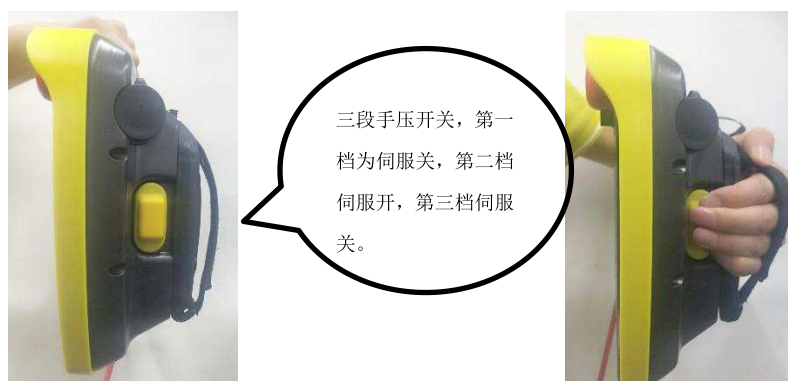
图 4.6.11 示教器握持方法
