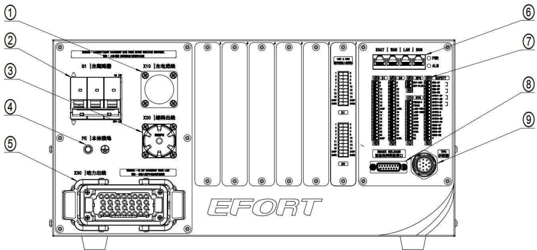
图 2.2.1 部件信息
