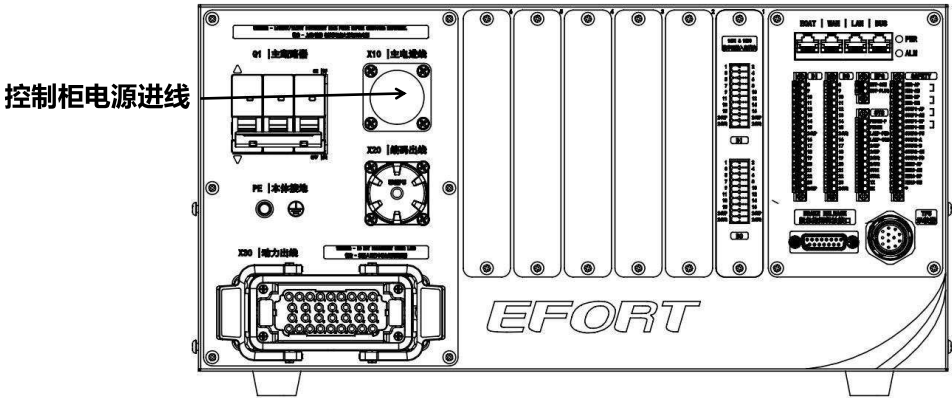
图 4.2.4 控制柜电源插头位置
