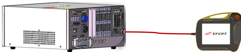
图 4.3.4 示教器电缆连接示意图
