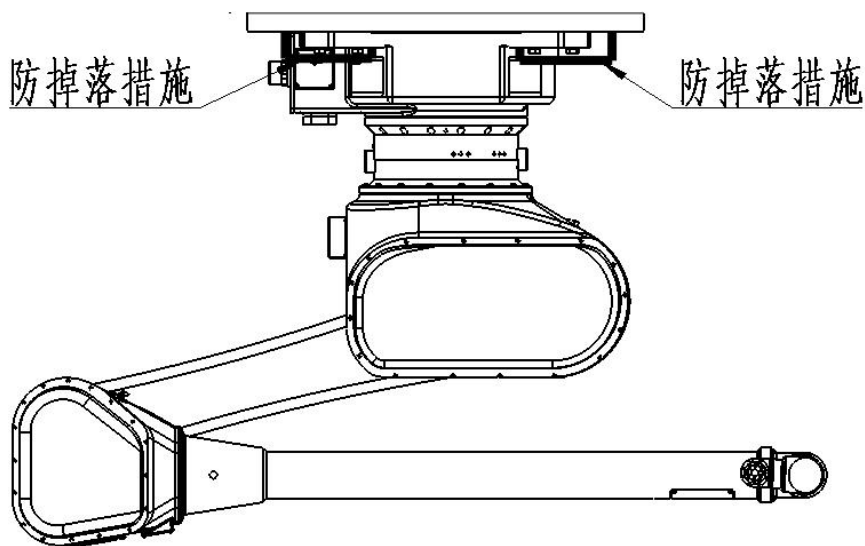
图 3-5 壁挂/倒挂安装
