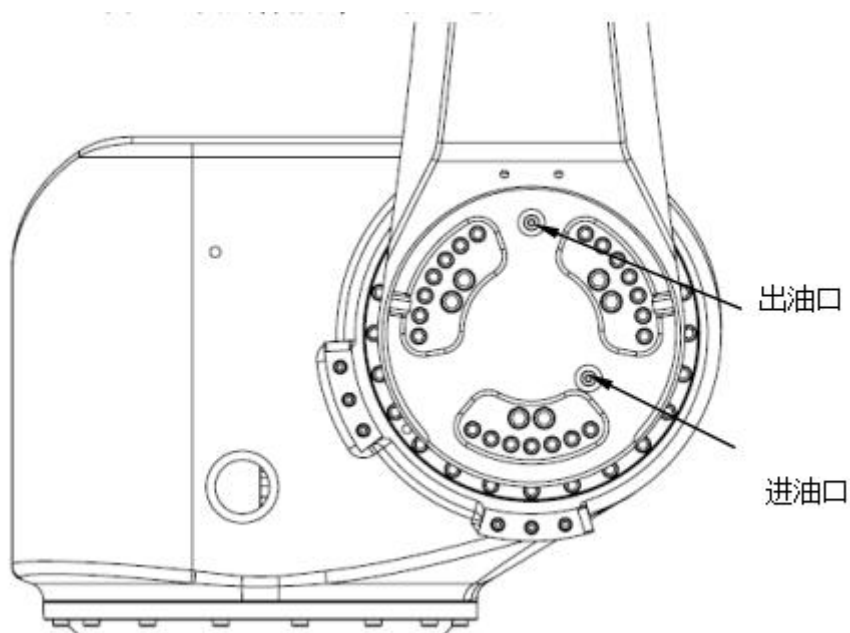
图 4-1 更换润滑油, J1 轴减速机
