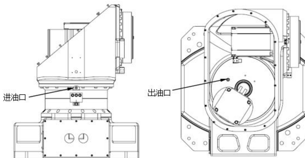
图 4-1 更换润滑油, J1 轴减速机
