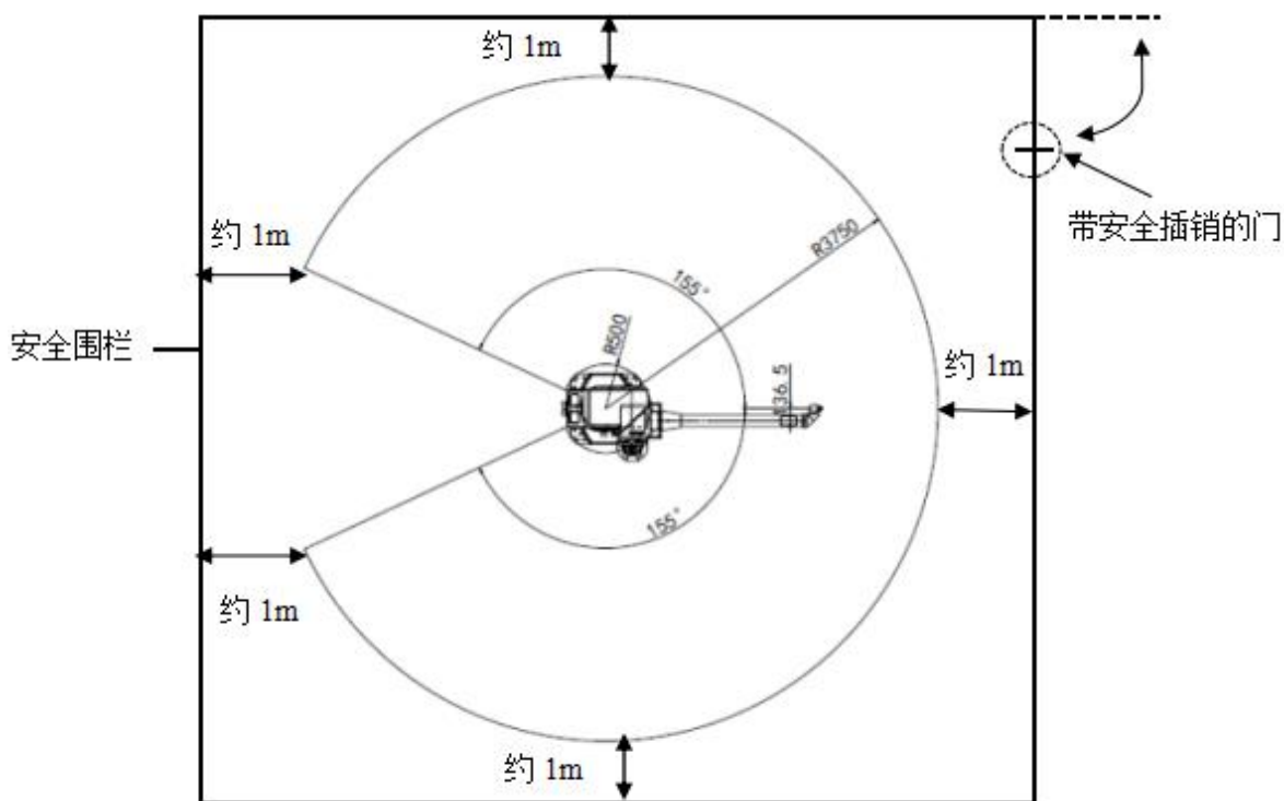
图 4-6 维护及使用区域
