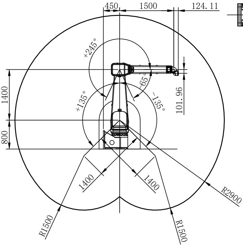
P点运动范围图 Point P locus
