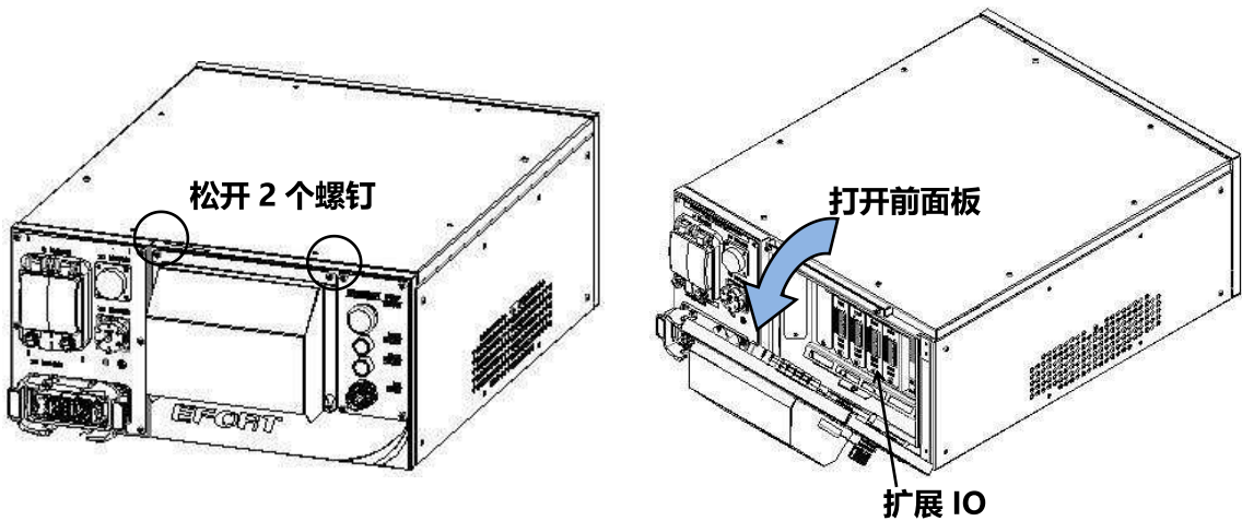
图 4.4.11 扩展 IO 位置示意图
