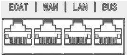
图 4.6.3 网络接口图示
