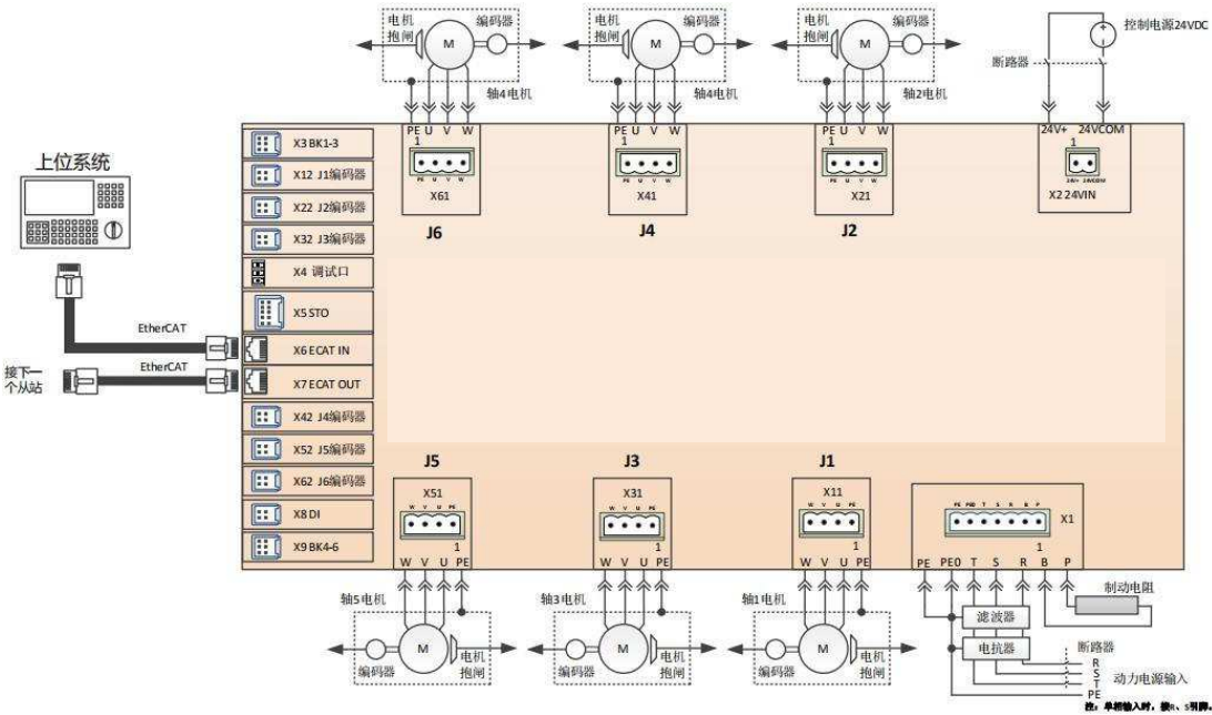
图 4.4.1 6 轴驱动器接线图
