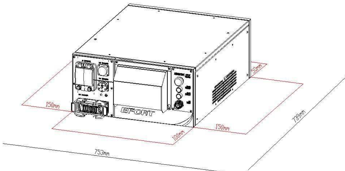
图 2.2.3 EC2-S (IP54) 控制柜所需安装尺寸
