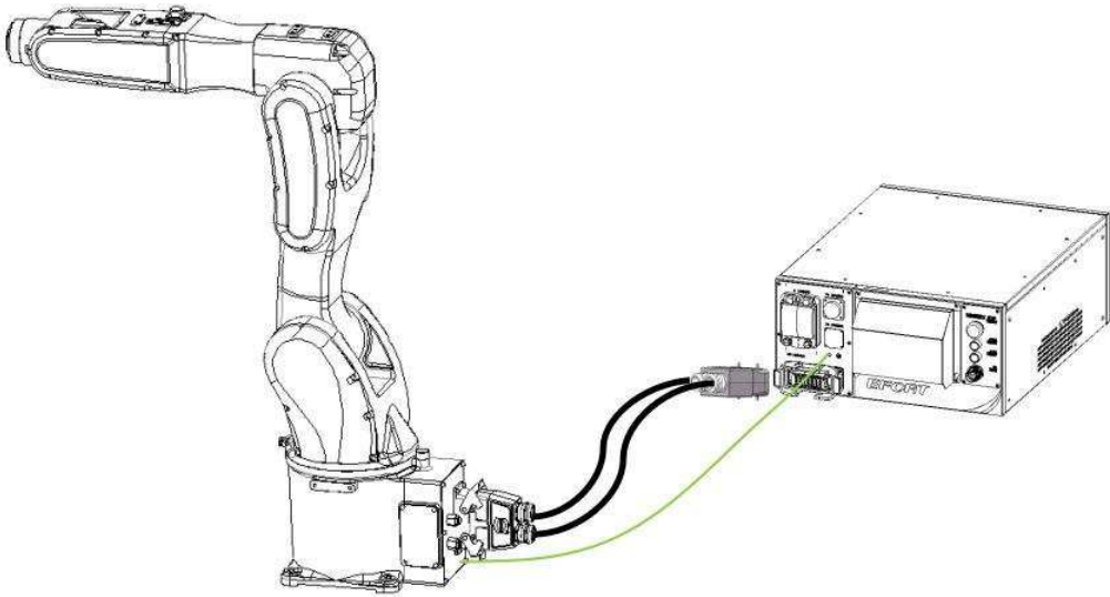
图 4.3.2 航插器电缆连接示意图
