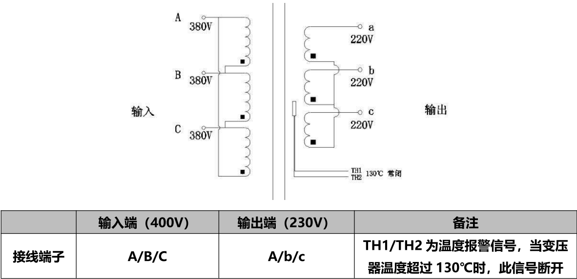
图 4.7.2 变压器接线图：
