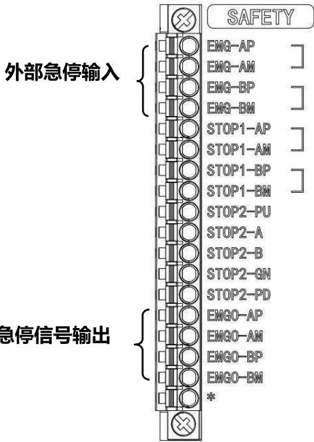
图 4.6.4 急停功能接线图
