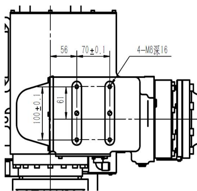
图 3-10 电机座上安装外部件尺寸图
