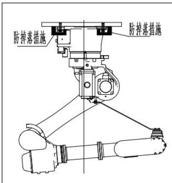
图 3-7 倒挂安装示例
