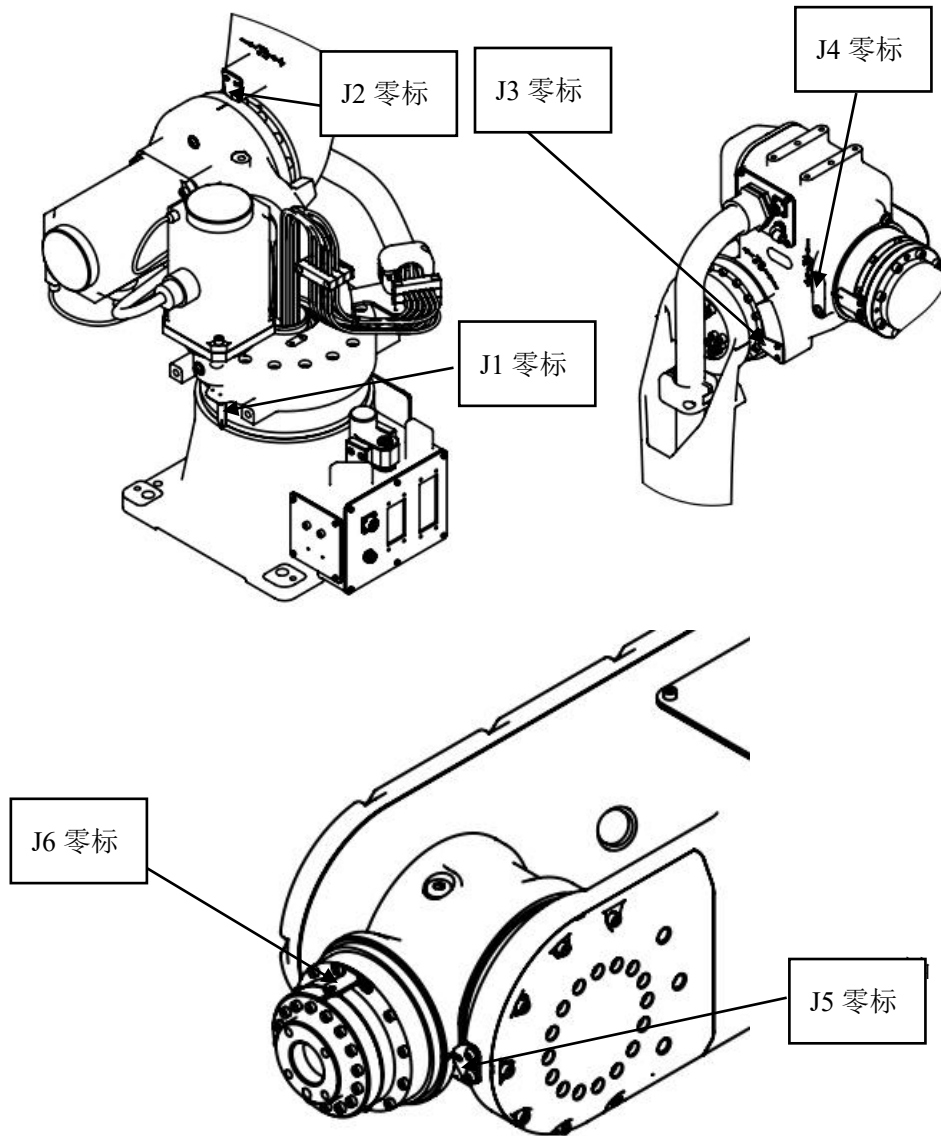
图 4-5 机器人零点位置图
