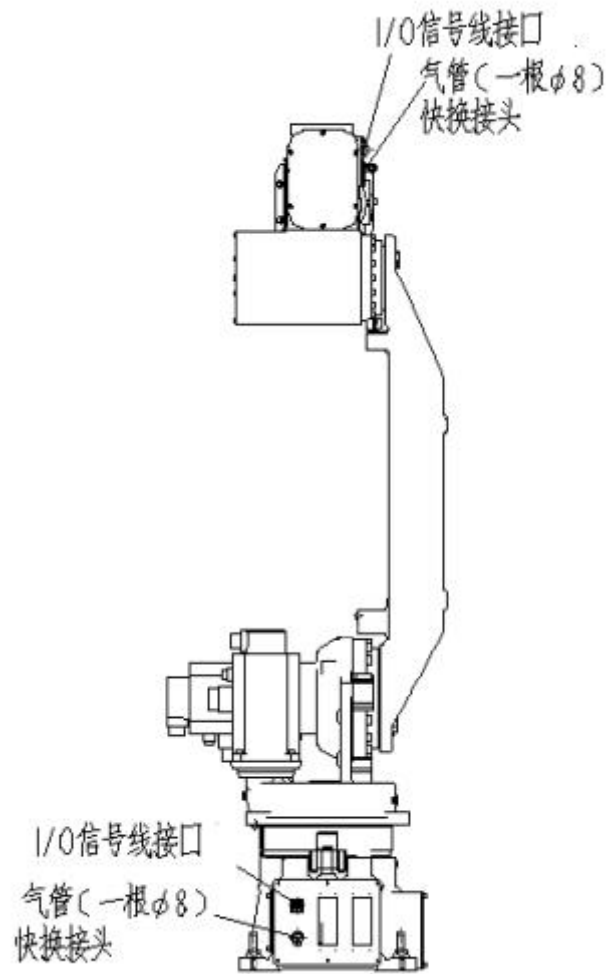
图 3-11 外接气管和信号线
