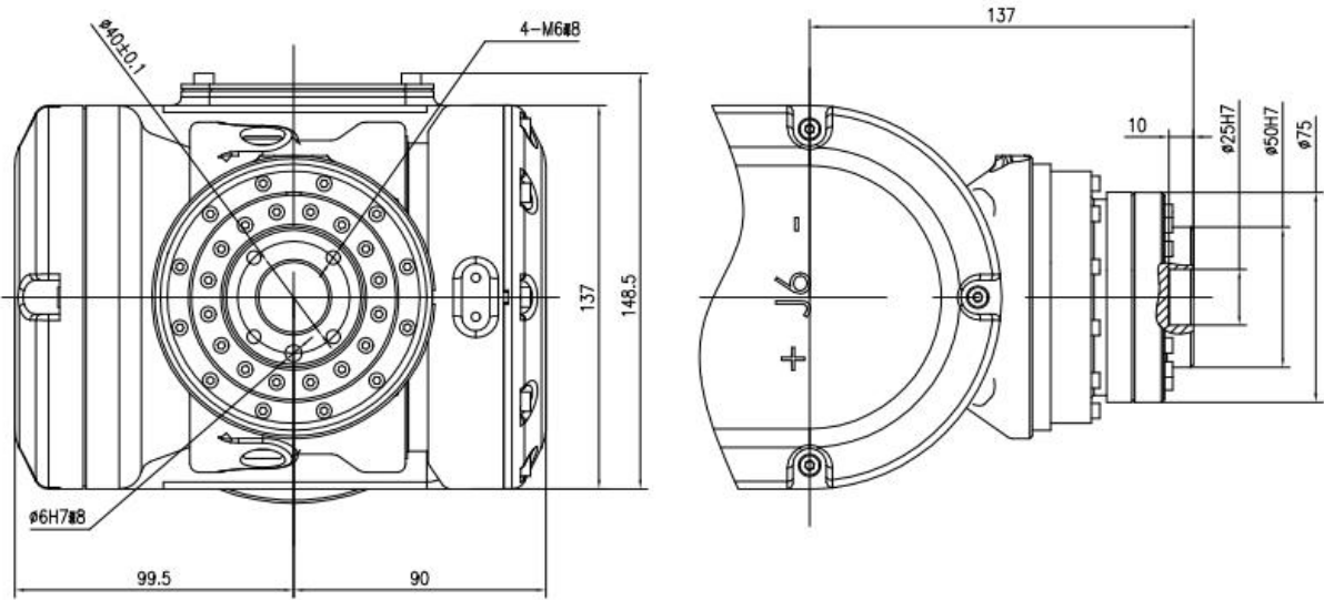
图 3-8 末端负载安装法兰尺寸
