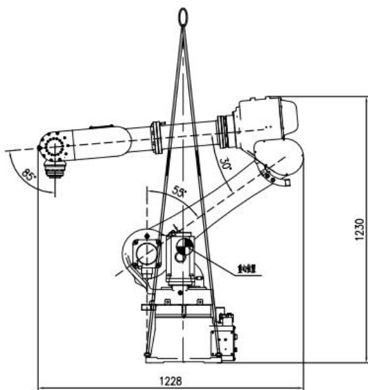
图 3-3 ER10-2000 吊装搬运示意图
