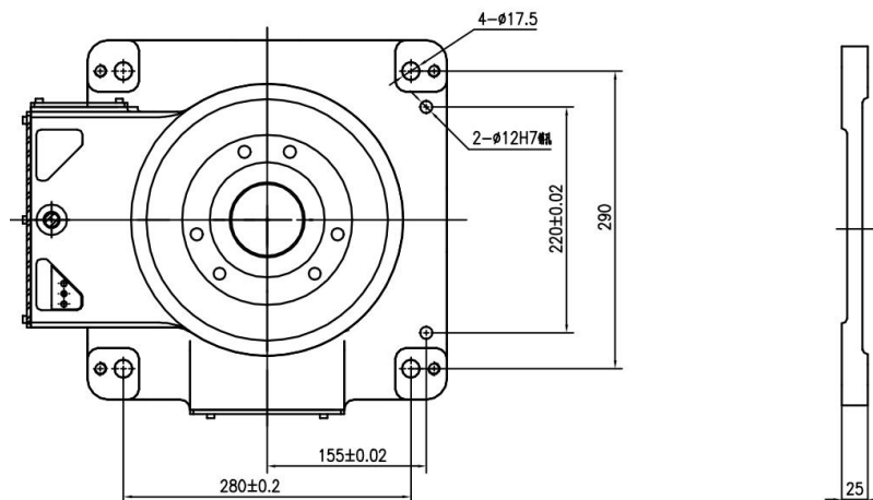
图 3-5 机器人底座尺寸
