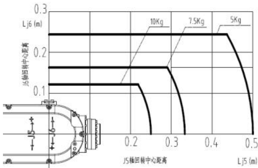
图 2-6 ER20-2000 手腕轴扭矩图
