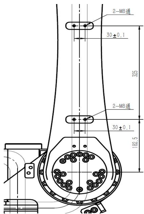
图 3-9 大臂上安装外部件尺寸图
