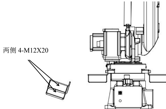
图 3-2 叉脚安装示意图
