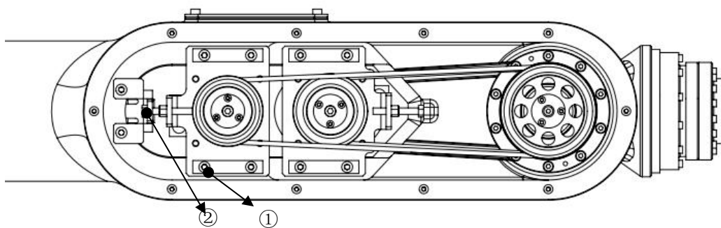
图 4-2 ER10-2000 机器人 J5 轴同步带结构图
