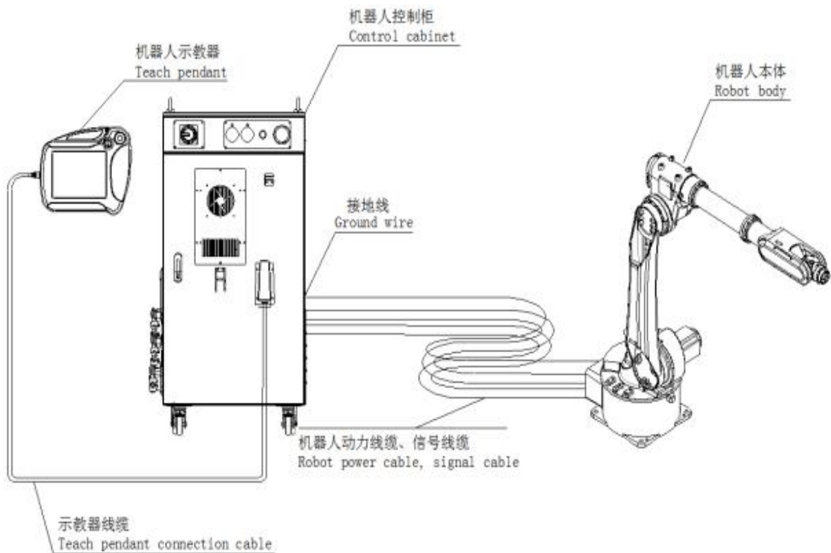
图 2-1 工业机器人系统构成
