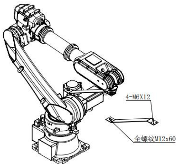
图 3-1 打包固定支架安装示意图
