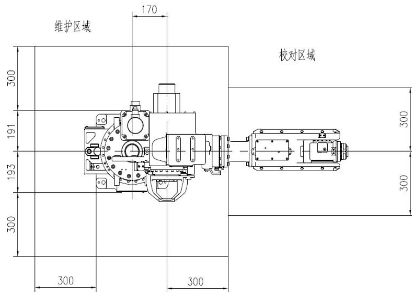
图 4-4 维护及使用区域
