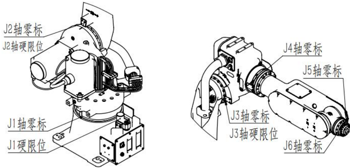
图 2-4 机械硬限位位置及零标位置
