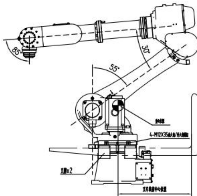
图 3-4 ER10-2000 叉车搬运示意图
