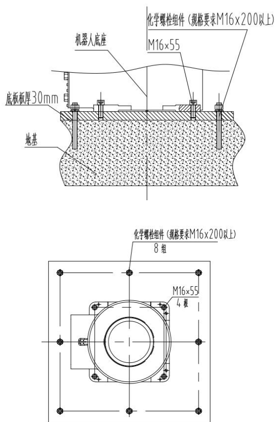
图 3-6 “机器人安装举例”
