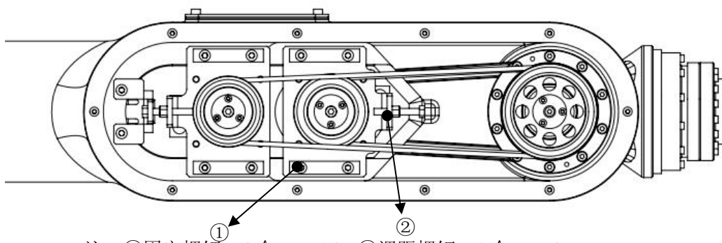
图 4-3 ER10-2000 机器人 J6 轴同步带结构图
